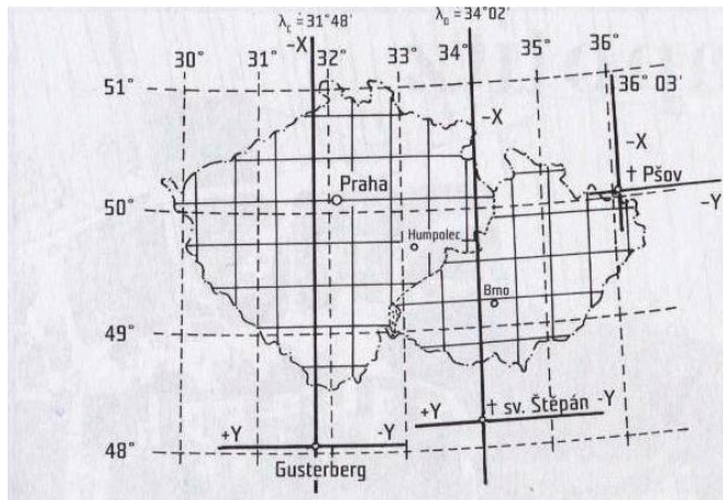
Obr. č. 1 – souřadnicová soustava stabilního katastru (Maršíková et Maršík, 2007)
