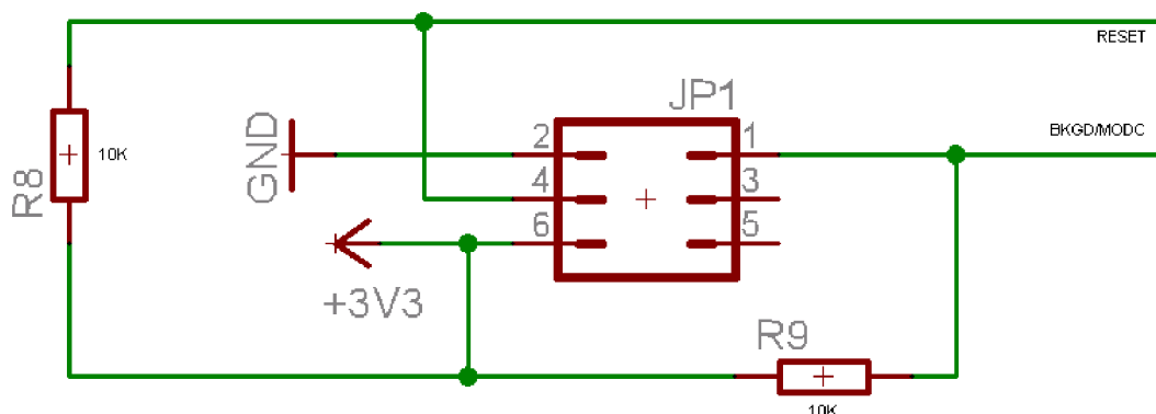
Obrázek 4.8 Schéma zapojení BKGD
