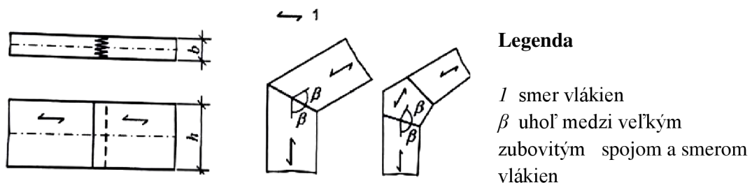
Obrázok č. 9 Veľké zubovité spoje v nosniku a rámovom rohu [7]
