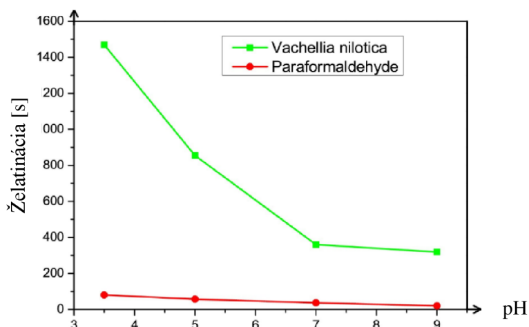
Obrázok č. 15 Porovnanie želatinácia pri rôznych pH lepidiel na báze tanínu s tvrdidlom paraformaldehydom a s tvrdidlom v podobe exsudátu z kôry afrického stromu Vachellia nilotica [22]
