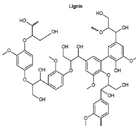
Obrázok č. 13 Štruktúra lignínu [18]
