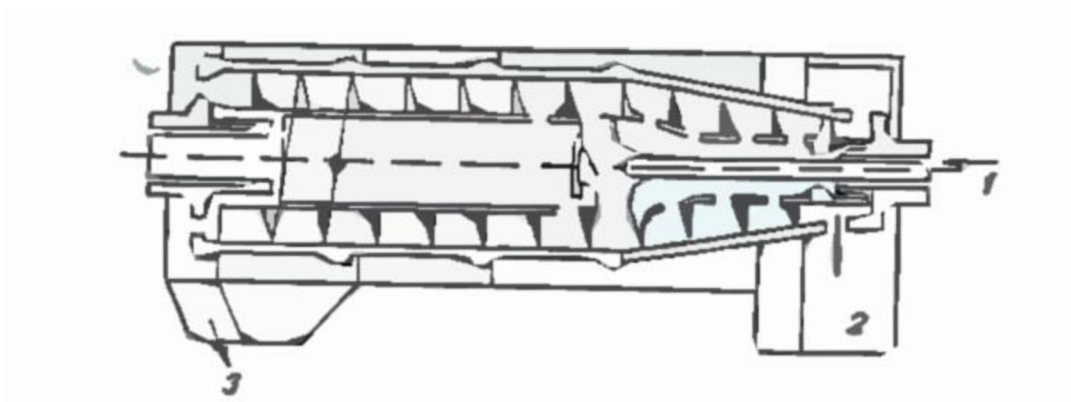
Obr. 7 Schéma odstředivky [23]
