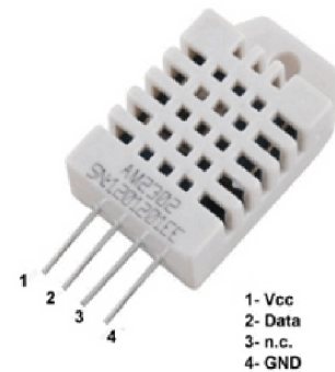
Obr. 5: Snímač teploty a vlhkosti DHT22[11]
