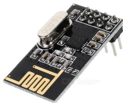
Obr. 3: Bezdrôtový modul nRF24L01+[14]
