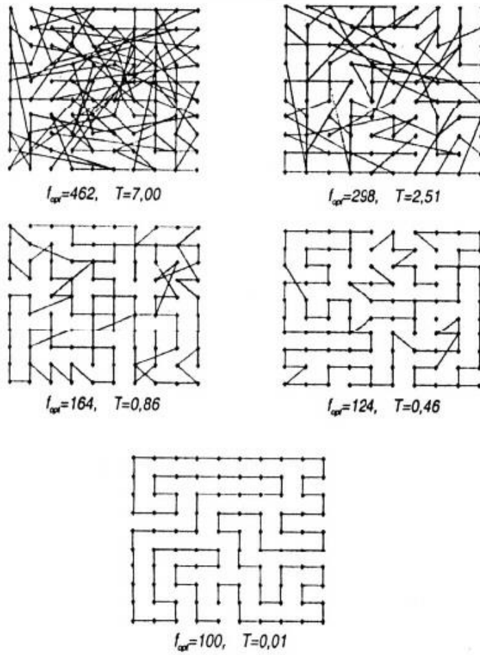
Obrázok 2.4: Simulované žhanie – postupné znižovanie teploty (zdroj: KENDALL a kol, 1999)
