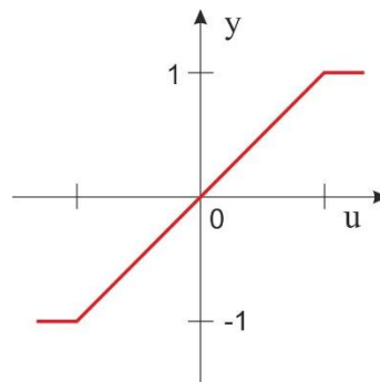
Obrázok 2.7: Čiasťočne lineárna prenosová funkcia
