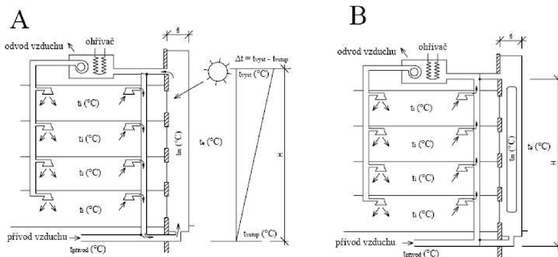
Obr. 7 Schéma budovy s dvojitou transparentní fasádou s meziprostorem šířky \delta a výšky H [m], která je totožná s výškou budovy, tj. 4 podlaží. Pohyb vzduchu je nucený a z hlediska fyzikální podstaty meziprostoru se jedná o fasádu s uzavřeným okruhem v zimním období [2].
