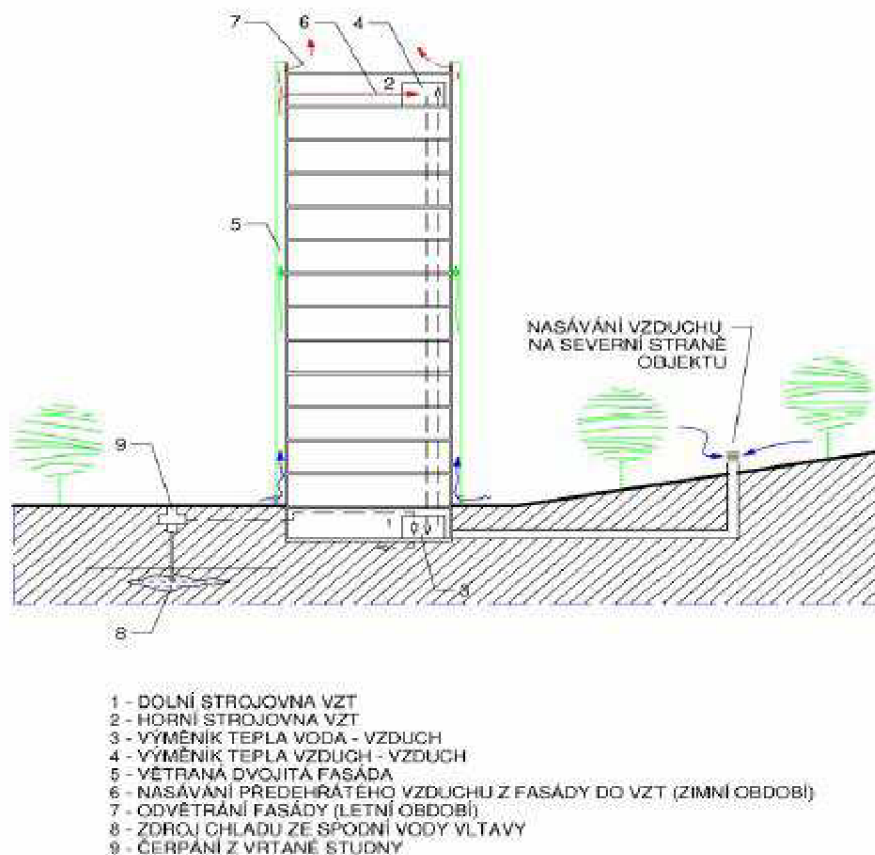
Obr. 21 Schéma teplovzdušného vytápění a větrání budovy využívajícího funkce dvojité hybridní solární fasády [13].
