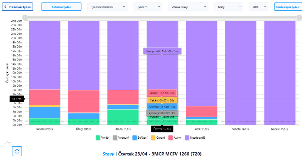
Obr. 32: Záznam týdenní aktivity stroje MCFV 1260 [64]
