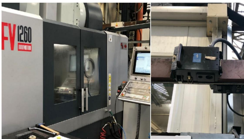
Obr. 15: Znáornění činnosti čištění průhledných bezpečnostních výplní pomocí obrázků
