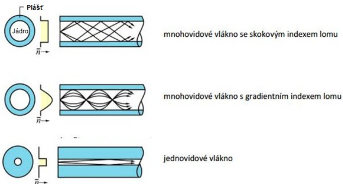
Obrázek 3: Optická vlákna dle vidů [12]
