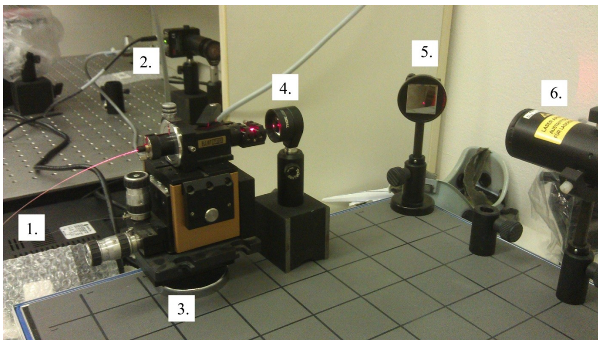
Obrázek 13: Optické pracoviště
