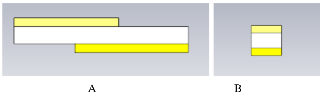
Obr. 14: Schematický náčrtek osamocené pásky, mezi jehož plochami vzniká laditelná kapacita. Kapacita je soustředěna především v dielektriku mezi sdíleným prostorem elektrod. (A) Nárys součástky – žluté pásy symbolizují měděné vodiče, bílá vrstva izolaci-dielektrikum, (B) bokorys součástky.
