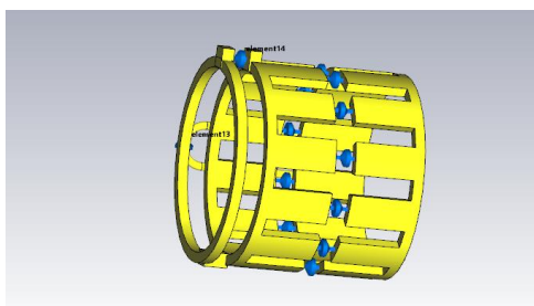
Obr. 11 a: Pohled na obvyklý způsob konstrukce ladění birdcage cívky a simulaci pole promítnutou na řezu
