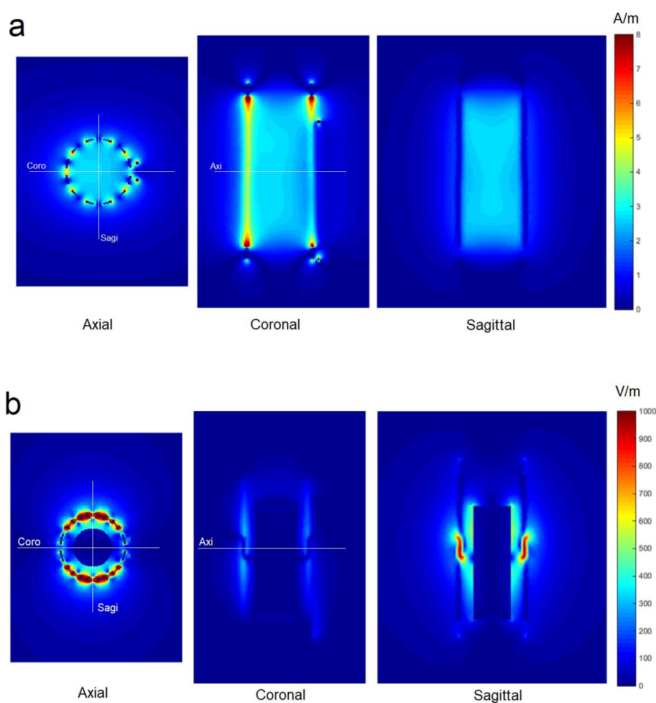
Obr. 21: Simulace magnetického pole v ^1\text{H}/^{19}\text{F} cívce se zátěží (50 ml váleček izotonické vody) (a), Simulace elektrického pole v ^1\text{H}/^{19}\text{F} cívce (50 ml váleček izotonické vody); Převzato z publikace [38]
