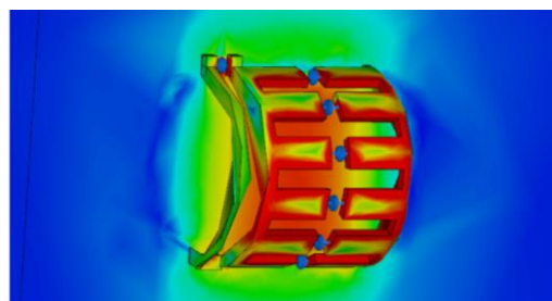
Obr. 11 a: Pohled na obvyklý způsob konstrukce ladění birdcage cívky a simulaci pole promítnutou na řezu
