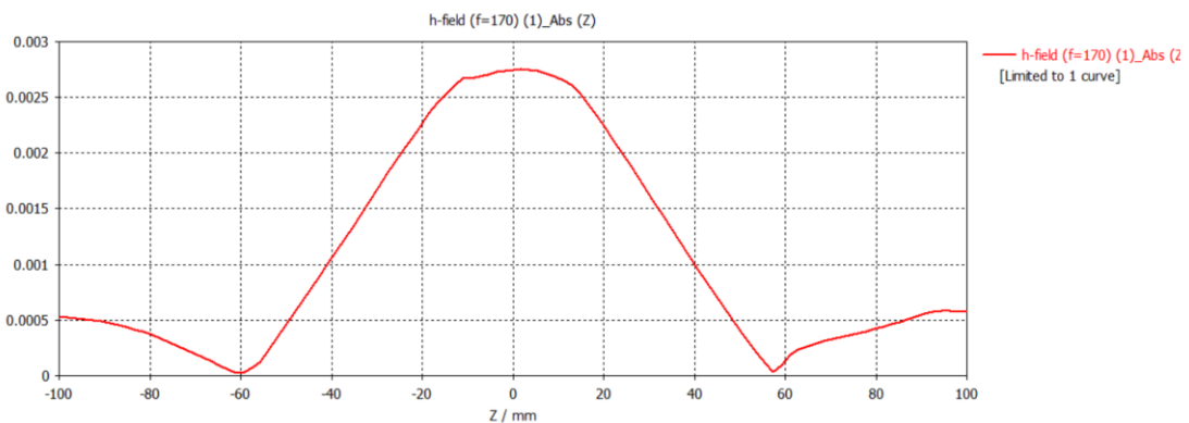
Obr. 9 b: Sagitální rozložení pole s vynesím intenzity magnetického pole v 1d grafu. Koordináty os: Z[-100,100], X[0], Y[0]. Intenzita mag. pole ve vakuu je vypočtena ze složek vektorů užitečných pro MR jako
