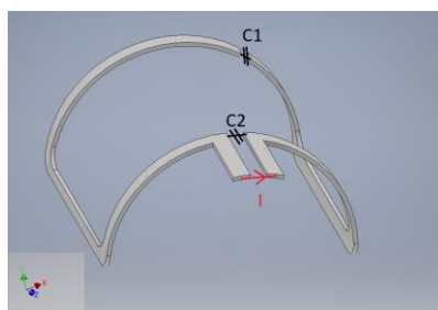
Obr. 8 a: Half-saddle radiofrekvenční cívka
