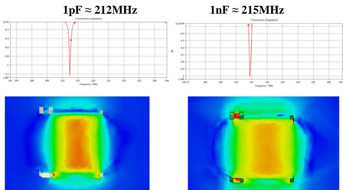
Obr. 11 b: Rozdílné nastavení ladicího kondenzátoru 1pF/1nF a způsobená změna rezonanční frekvence cívky spolu se změnou distribuce RF pole
