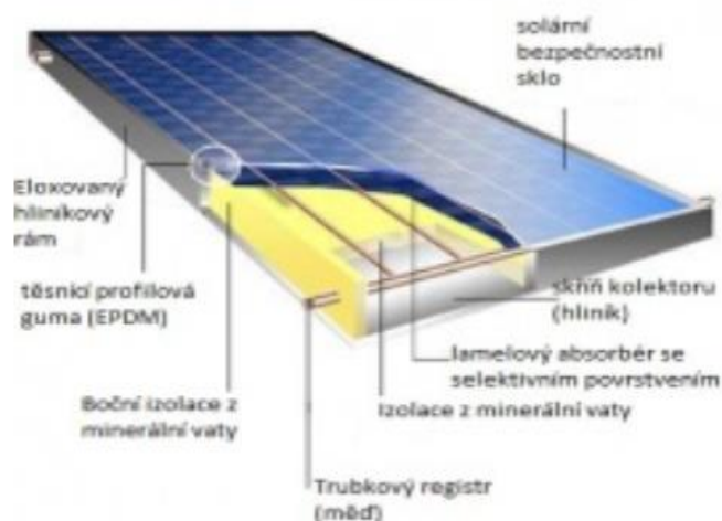
Obrázek 6 Konstrukce solárního kolektoru
