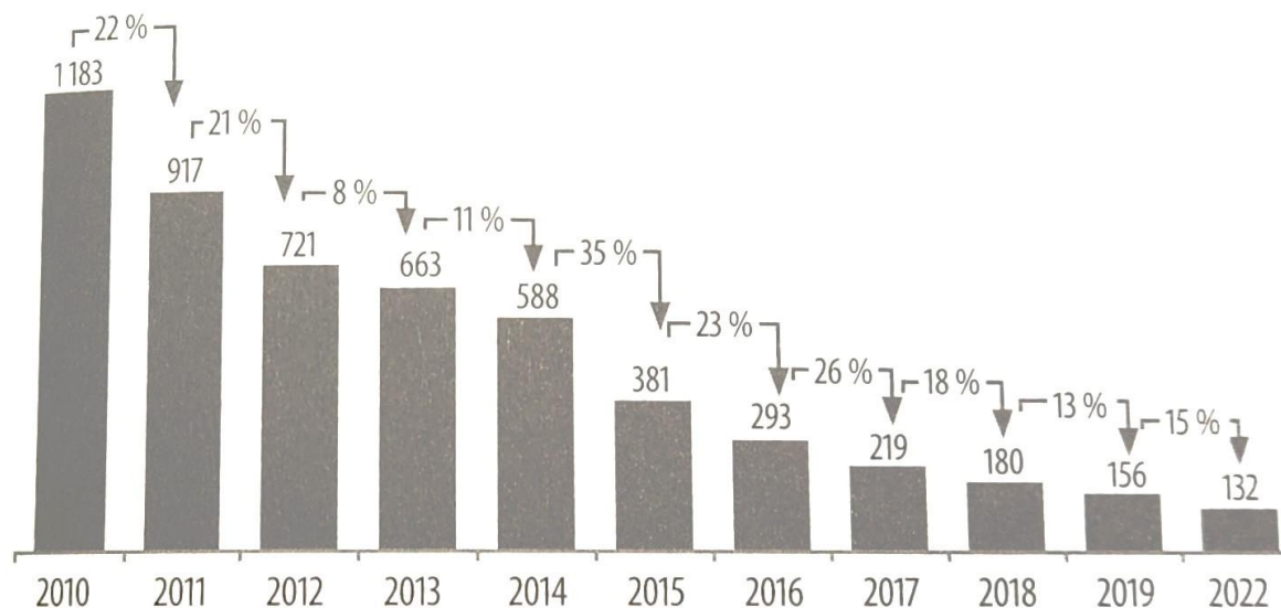
Graf 2 Vývoj cen baterii v USD za kWh
