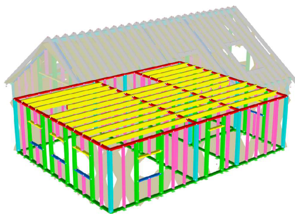
Obrázok 4 Prvky prízemnia
