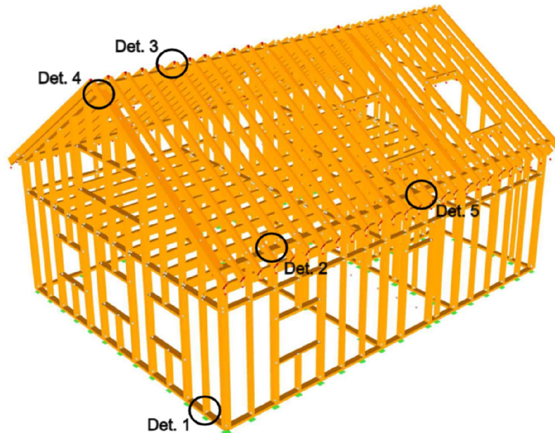
Obrázok 16 Umiestnenie spojov
