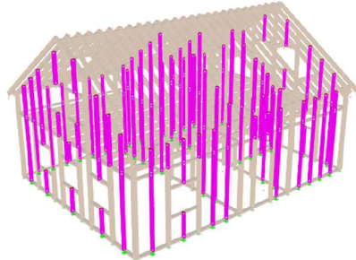
Obrázok 7 Stĺpiky 60/140
