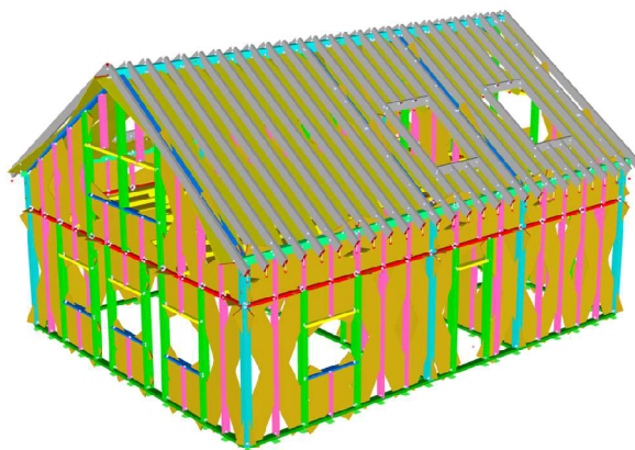
Obrázok 3 Model konštrukcie vrátane fiktívnych prútov
