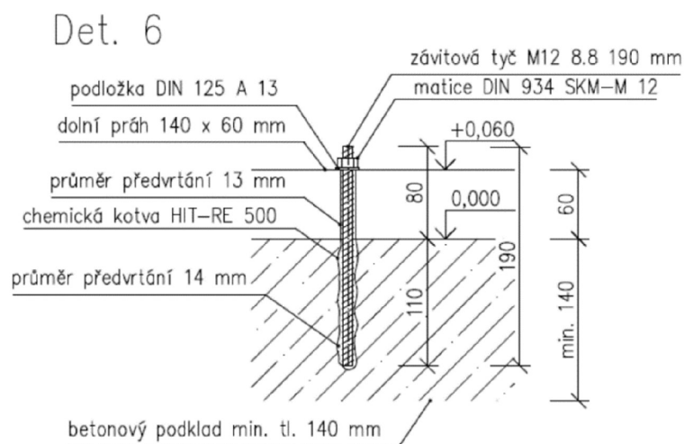
Obrázok 17 Detail kotvenia
