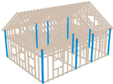
Obrázok 8 Rohové stĺpiky 140/140
