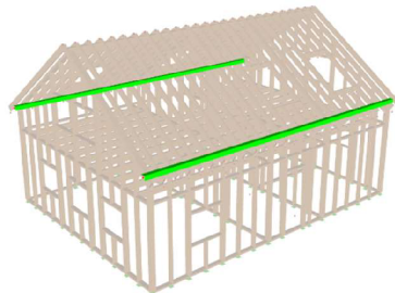
Obrázok 13 Väznica 140/140
