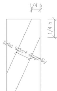
Obrázok 14 Fiktívny prút
