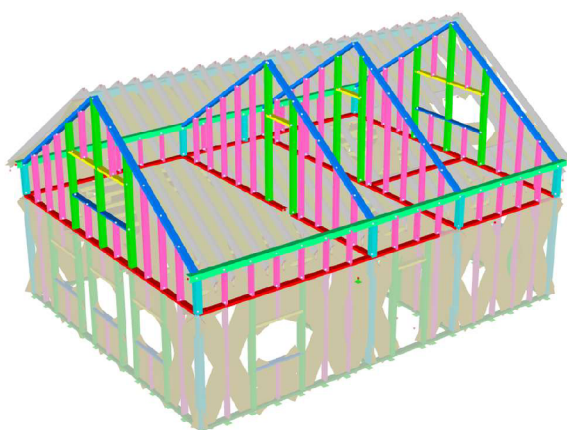
Obrázok 5 Prvky podkrovia
