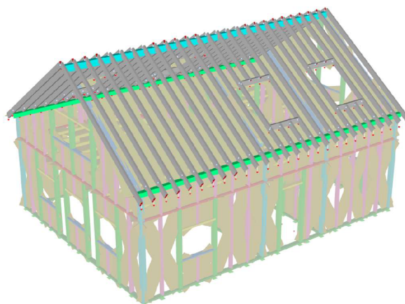
Obrázok 6 Prvky krovu
