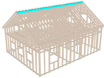
Obrázok 12 Vrcholová väznica 140/200
