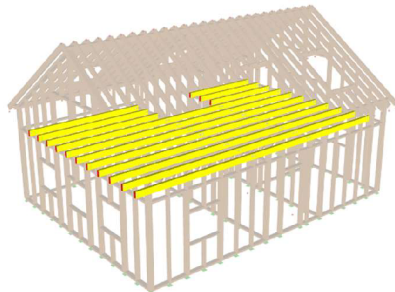
Obrázok 10 Stropné trámy 80/200
