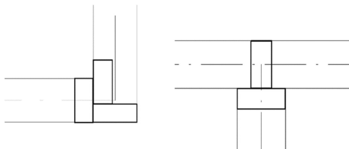
Obrázok 9 Skutočné usporiadanie stĺpikov v rohu
