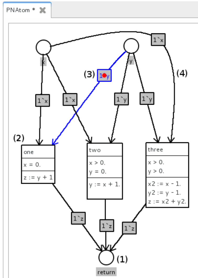
Obrázek 7.12: Model vytvořený pomocí Petriho sítě.
