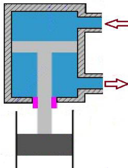
Obr. 23 Hydraulický lis [9]
