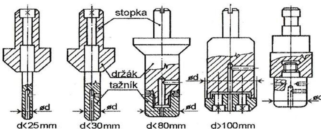
Obr. 20 Konstrukce tažníku [7]
