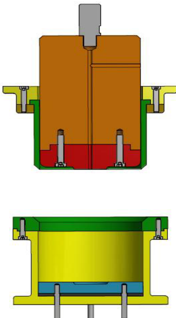
Obr. 29 Nástroj
