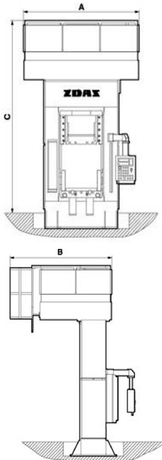
Obr. 33 Stroj [10]
