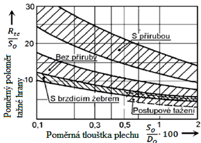
Obr. 19 Graf ke stanovení R_{tc} [7]
