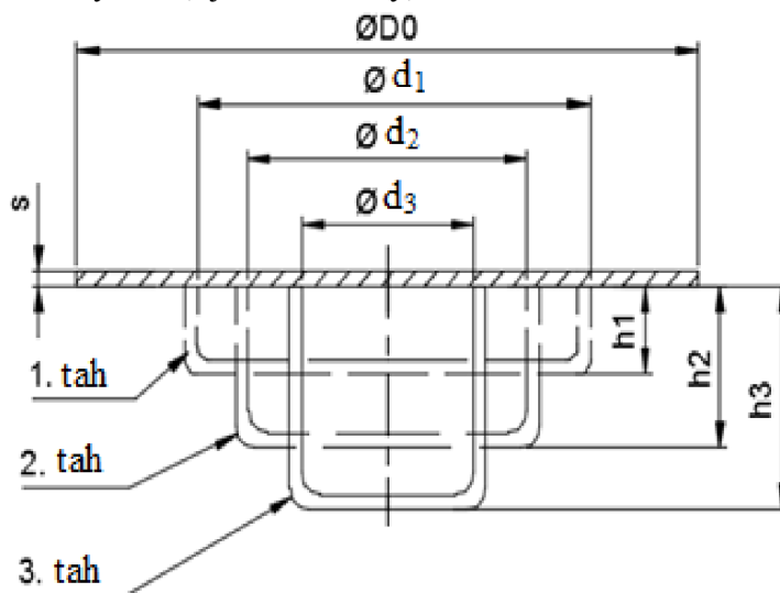
Obr. 14 Tažné operace [20]
