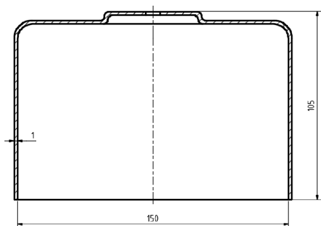
Obr. 3 Kryt vzduchového filtru
