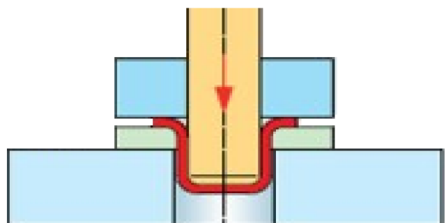
Obr. 8 Konvenční tažení [4]
