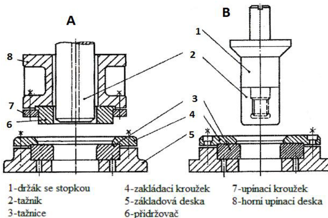
Obr. 17 Tažný nástroj [7]
