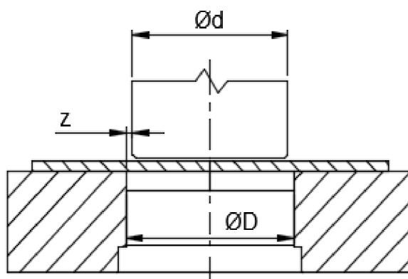
Obr. 15 Tažná mezera [30]
