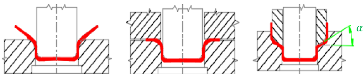
bez přidržovače
