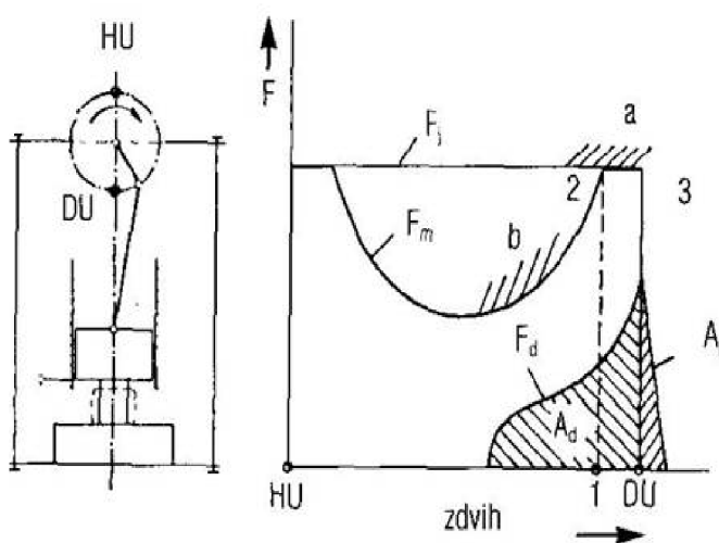
Obr. 22 Mechanický lis [26]
