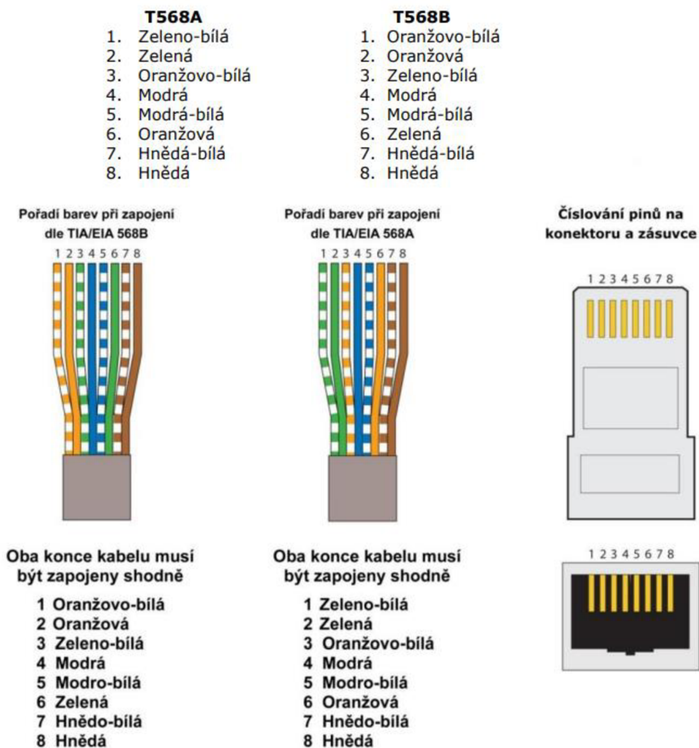
Obrázek 6 Zapojení kabeláže dle standartu TIA/EIA [7]
