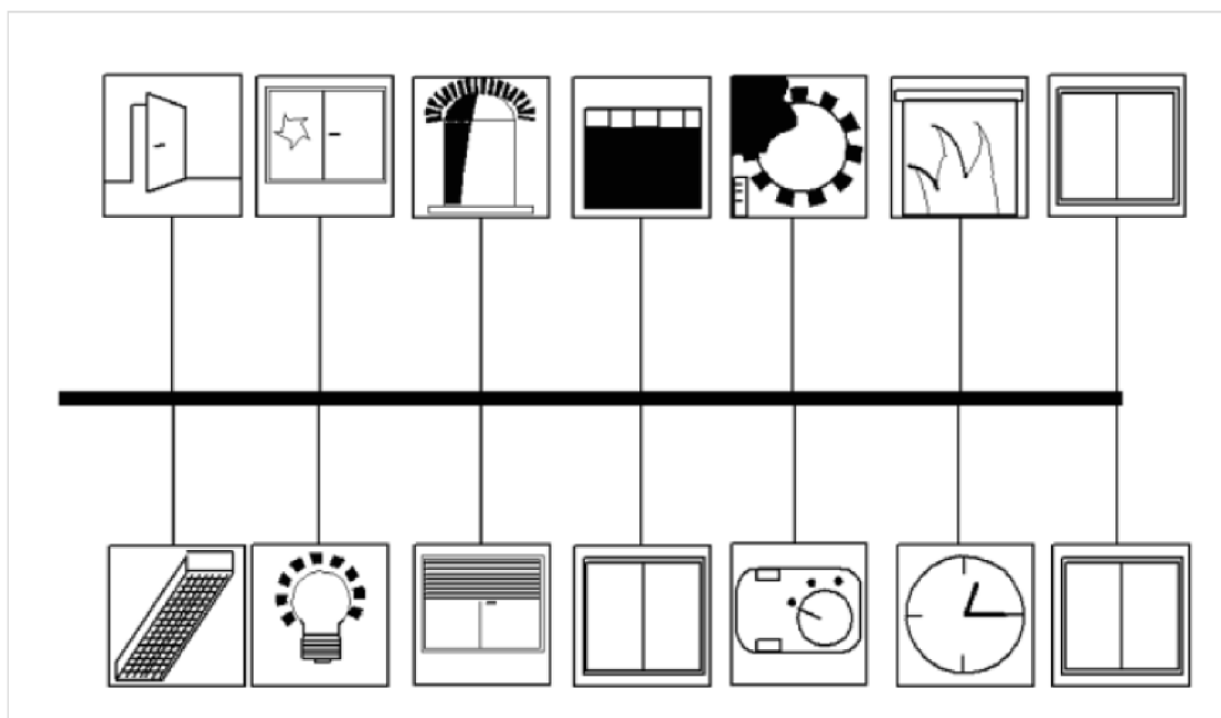
Obrázek 8 Sběrníková instalace [14]
