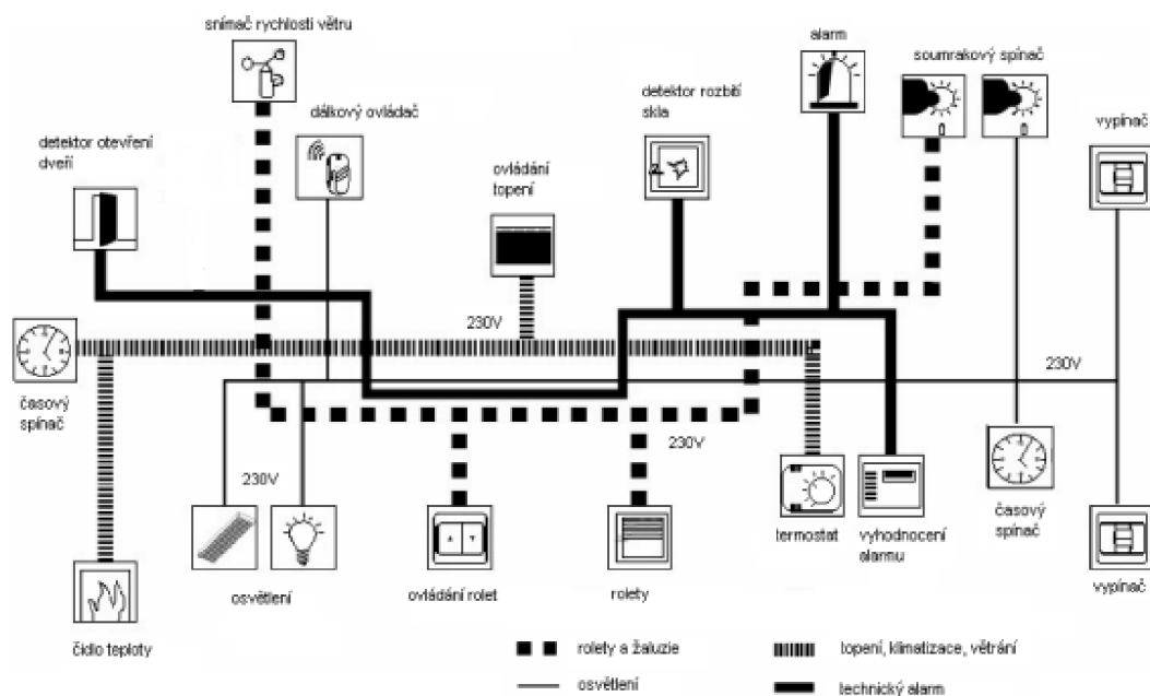
Obrázek 7 Klasická instalace [14]
