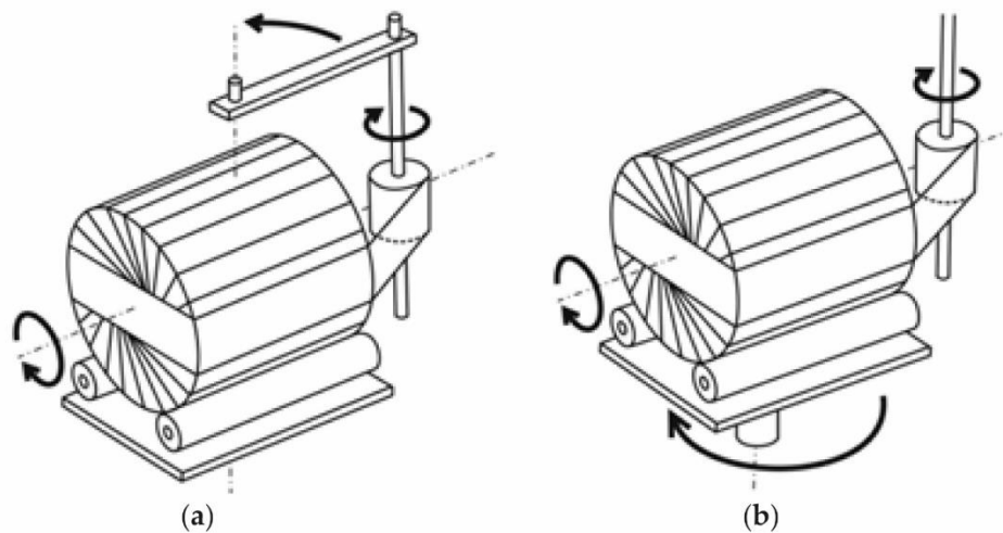
Obr. č. 15 Základní typy provedení ovíječek Zdroj: STANKIEWICZ, 2019
