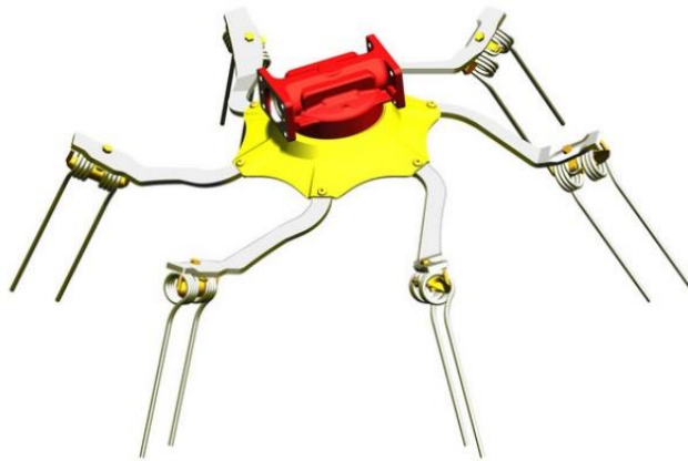
Obr. č. 6 Rotor obraceče s inovovanými hrabícemi
