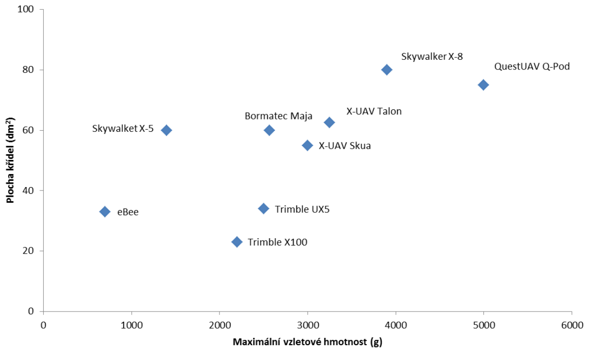
Graf 9 Závislost maximální vzletové hmotnosti na ploše křídel jednotlivých platform.
