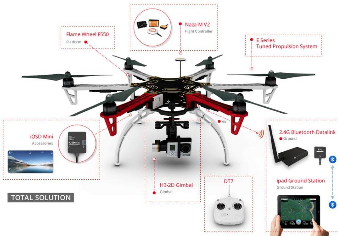
Obrázek 37 Vybavení hexakoptéry F550 všemi dostupnými prvky Nazi-M V2.
