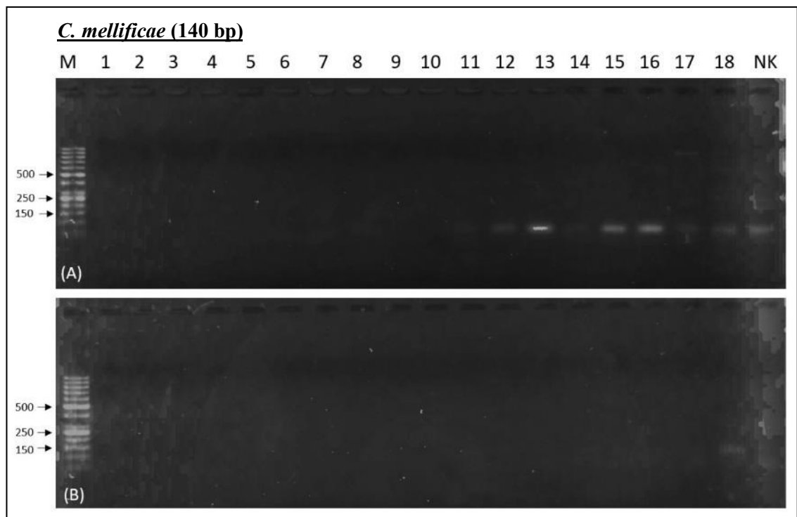
Obr. 23 Porovnání elektroferogramů produktů PCR pro detekci C. melliferae . (A) výsledky z DNA izolačního kitu Qiagen. (B) výsledky z FTA karet. M: marker GeneRuler 50 bp; 1-18: vybrané podzimní vzorky včel; NK: negativní kontrola.
