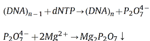
Obr. 7 Reakční schéma vzniku precipitátu při LAMP reakci. Převzato ze Zhang et al., 2014.
