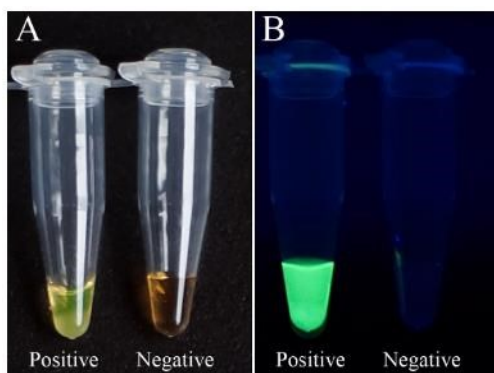
Obr. 9 Použití SYBR Green I pro vizualizaci LAMP produktů. A: zkumavky v přirozeném světle. B: UV záření. Převzato z Nie et al., 2012.
