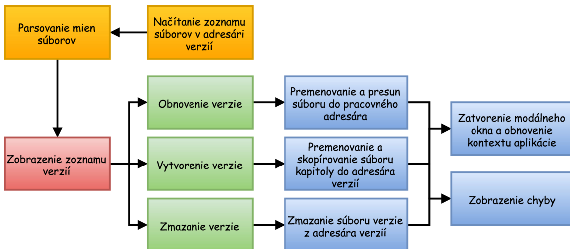
Obr. 3.23: Stavový graf pre správu verzií
