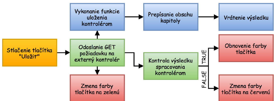
Obr. 3.22: Stavový graf pre ukladanie
