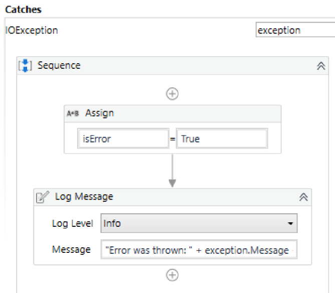
Obr. 5.1: Kód v bloku Catch
