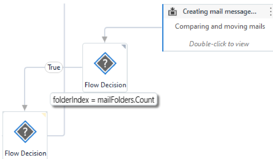
Obr. 5.20: Podmínka pro kontrolu další složky pro kategorizaci
