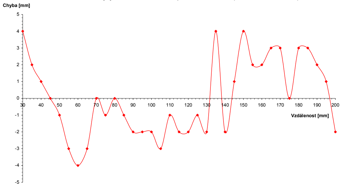
Grafická závislost chyby na měřené vzdálenosti pro dřevěnou desku (150mmx350mmx25mm)
