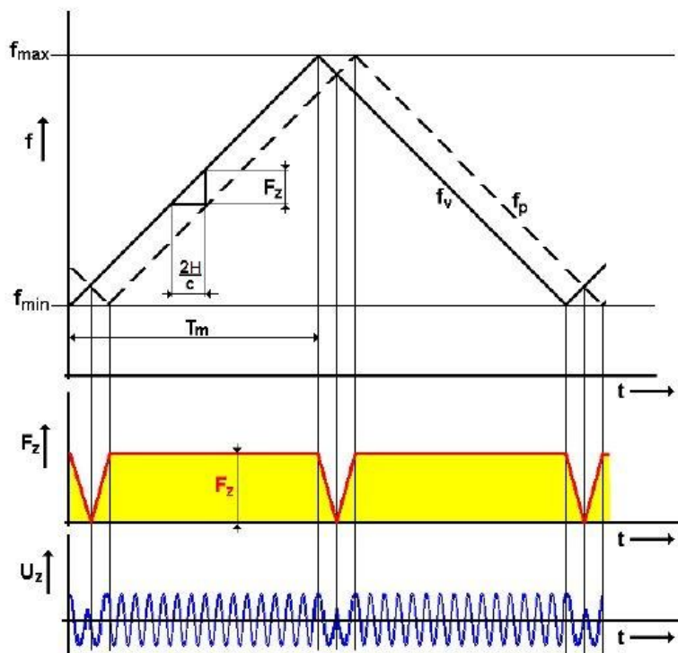
Obr. 13 Časové rozložení průběhů výškoměru, převzato z [5]
