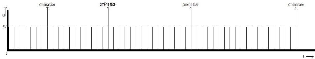
Obr. 14 Příklad posloupnosti vysílaného signálu o frekvenci
