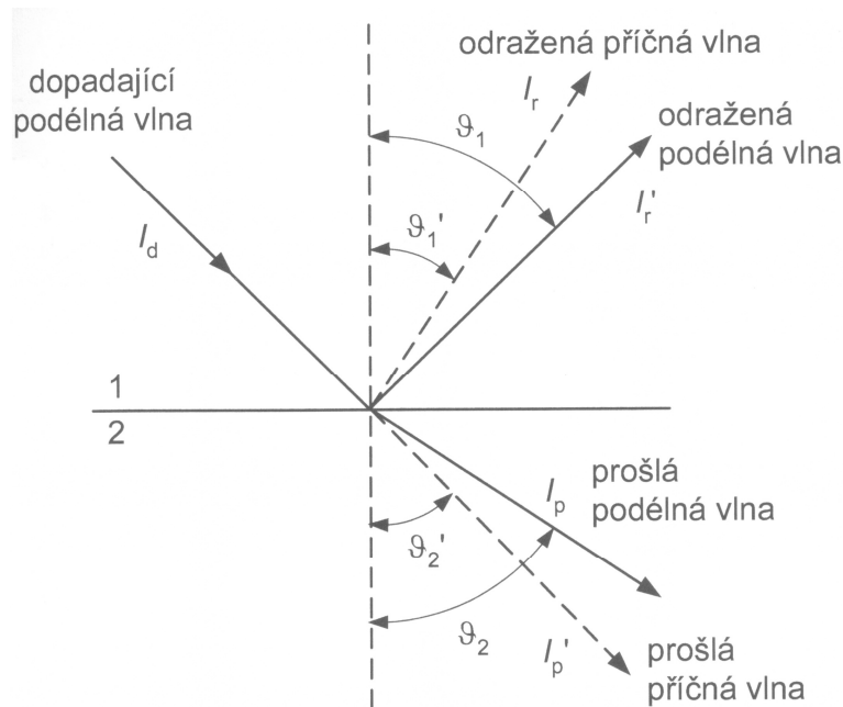
Obr. 3 Znáornění funkce lomu a odrazu, převzato z [1]
