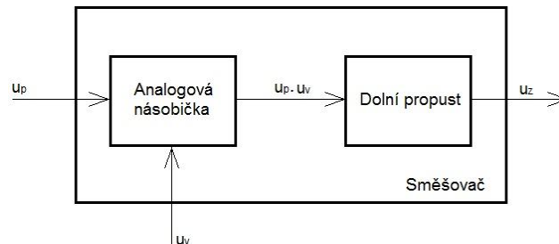
Obr. 12 Směšovač
