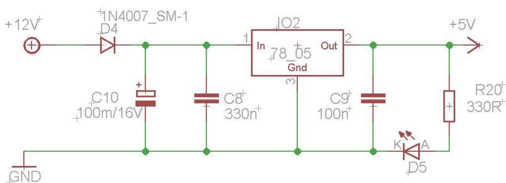
Obr. 44 Schéma napájecího bloku
