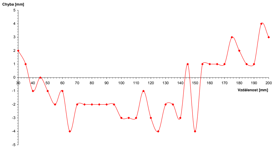
Grafická závislost chyby na měřené vzdálenosti pro betonovou dlaždici (170mmx500mmx40mm)
