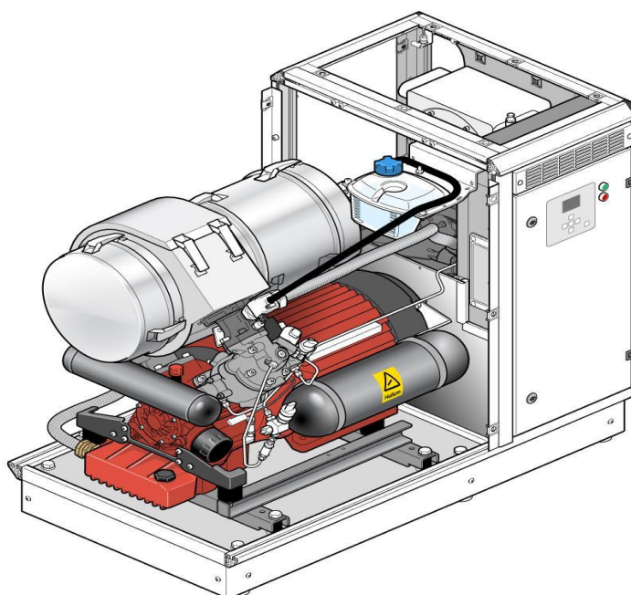
Obr. 26: Kogenerační jednotka společnosti Solo Stirling GmbH
