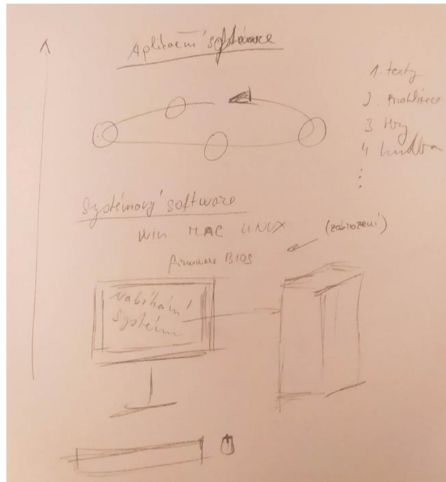
Obrázek 2- návrh software
