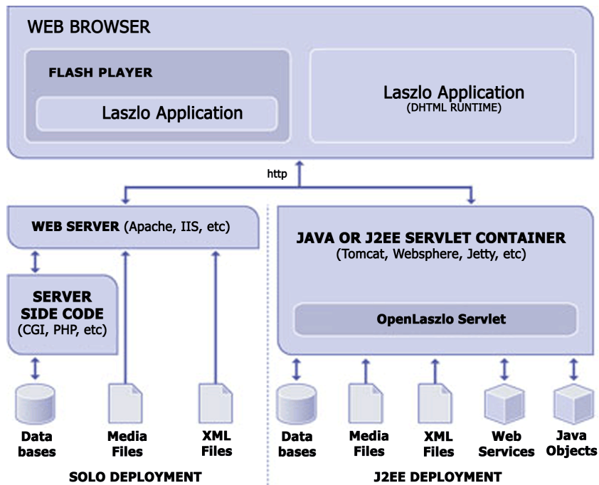
Obrázek 2.1: Architektura OpenLaszlo [14].
