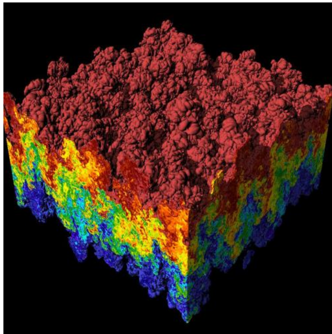
Obrázek 3.2: Ukázka moderní vědecké 3D vizualizace: Smíchání 2 tekutin [21].
