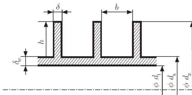
Obr. 6.4 Osový řez trubicou s kruhovými radiálními žebry ( d_i = d_1 , d_a = d_2 , d_z = d_{ze} ) [21]
