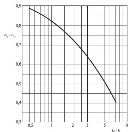
Obr. 6.5 Diagram závislosti poměru \alpha_{ze}/\alpha_0 na poměru h/b [21]
