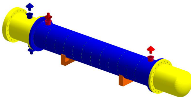
Obr. 5.1 3D náčrt výměníku tepla v HTRI Xchanger Suite 7.2 [9]
