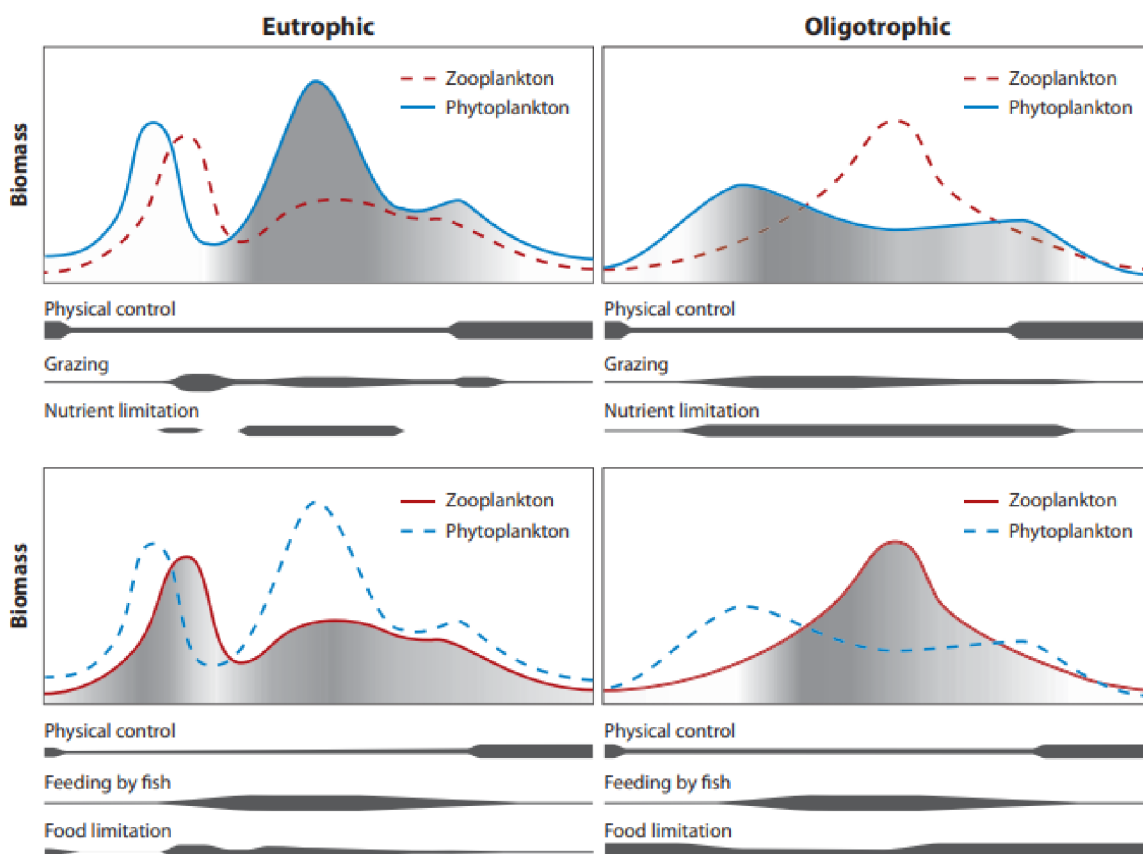
Obr. 1: Základní PEG model sezónního vývoje planktonu. Nalevo jsou uvedeny modely pro vývoj planktonu v eutrofních jezerech, vpravo v oligotrofních jezerech. Horní řádek modelů se zaměřuje na výskyt fytoplanktonu, kdy tmavě šedé zbarvení označuje koryši nevyžíráný fytoplankton, světlý odstín označuje vyžíráný fytoplankton. Dolní řádek modelů se zaměřuje na zooplankton, kdy tmavě šedé zbarvení označuje malé herbivory a světlý odstín označuje herbivory velké. Tloušťka horizontálních úseček označuje míru působení daného vlivu v daném období (zdroj: Sommer et al., 2012).
