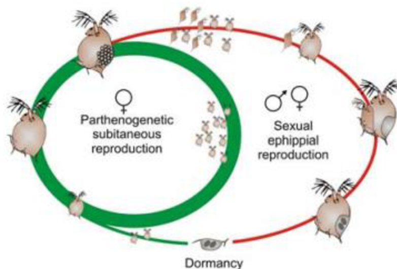
Obr. 2: Rozmnožovací cyklus (cyklická rodozměna) rodu Daphnia. Ve vhodných podmínkách se rozmnožují samice pomocí partenogeneze. Sexuální rozmnožování nastává při nevhodných podmínkách prostředí a důsledkem je trvalé vajíčko (zdroj: Decaestecker et al., 2009).
