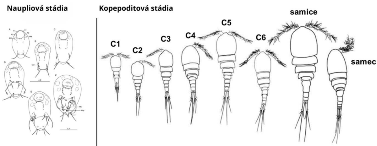
Obr. 3: Postembryonální vývoj klanonožce na ukázce Acanthocyclops robustus. Naupliová stádia jsou ukázána vlevo. Vpravo na obrázku jsou vyobrazena kopepoditová stádia, včetně dospělé samice a dospělého samce. Upraveno dle Bláhy, 2010 a Turki et al., 2002.
