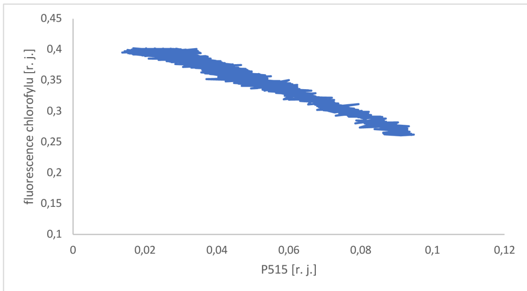
Obrázok 13: Závislosť fluorescence chlorofylu na signáli P515 pri intenzite 3000 \mu\text{mol} fotonov \text{m}^{-2} \text{s}^{-1} .
