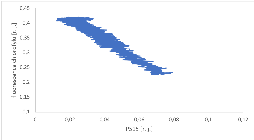
Obrázok 12: Závislosť fluorescence chlorofylu na signáli P515 pri intenzite 1000 \mu\text{mol} fotonov \text{m}^{-2} \text{s}^{-1} .
