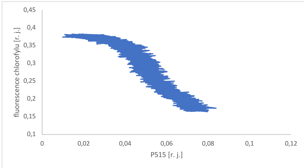
Obrázok 10: Závislosť fluorescencie chlorofylu na signáli P515 pri intenzite 300 \mu\text{mol fotónov m}^{-2} \text{s}^{-1} .
