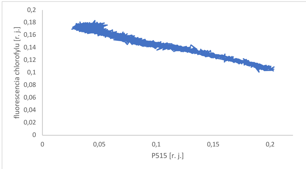
Obrázok 19: Závislosť fluorescencie chlorofylu na P515 pri izbovej teplote.
