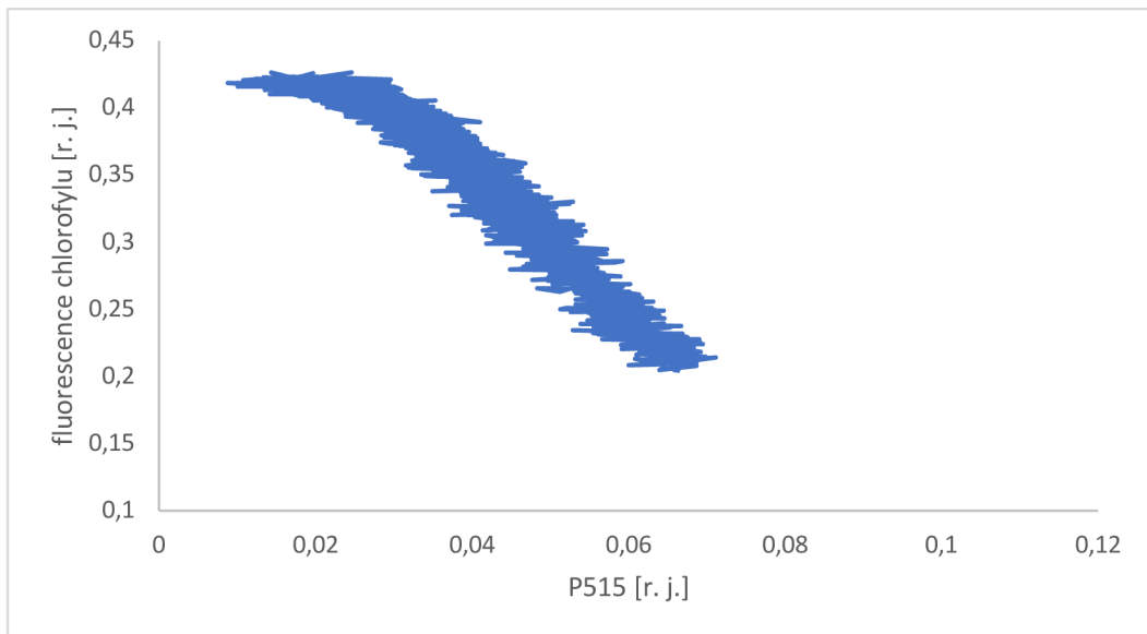
Obrázok 11: Závislosť fluorescencie chlorofylu na signáli P515 pri intenzite 500 \mu\text{mol fotónov m}^{-2} \text{s}^{-1} .
