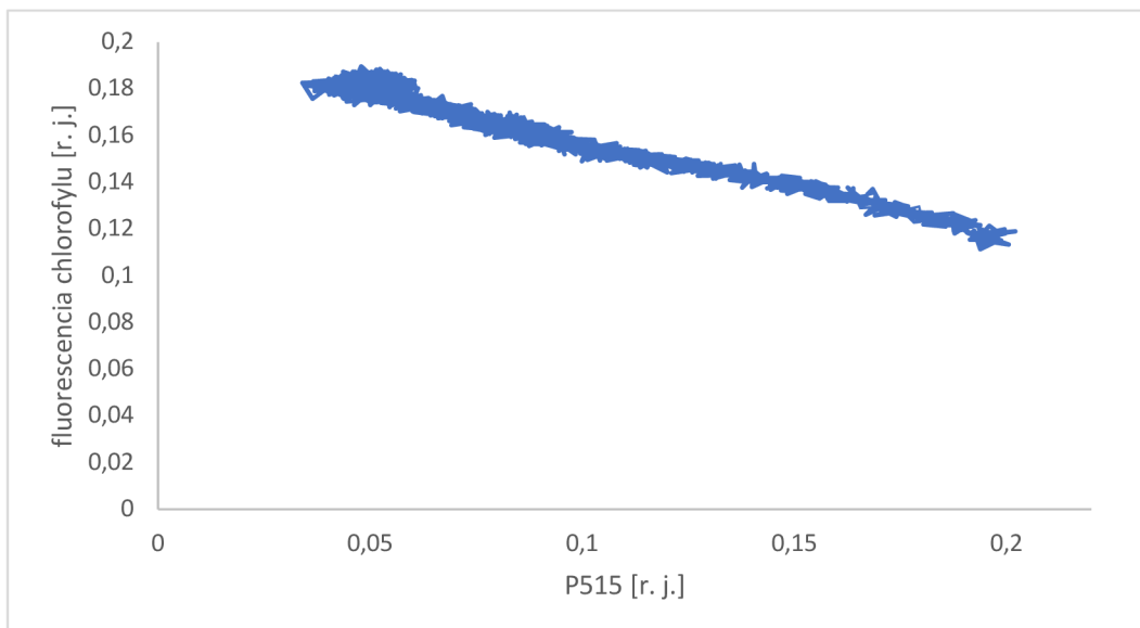
Obrázok 20: Závislosť fluorescencie chlorofylu na P515 pri 30°C.
