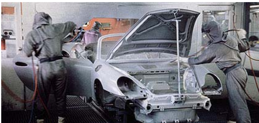
Obrázek 11: ruční nanášení plniče na karoserii Porsche boxer[9]
