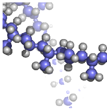
Obrázek 19: struktura polypropylenu
