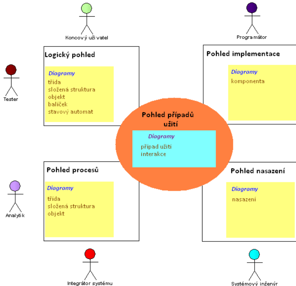
Obrázek 9 - Pohled 4+1
