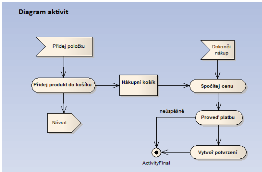
Obrázek 7 - Diagram aktivit
