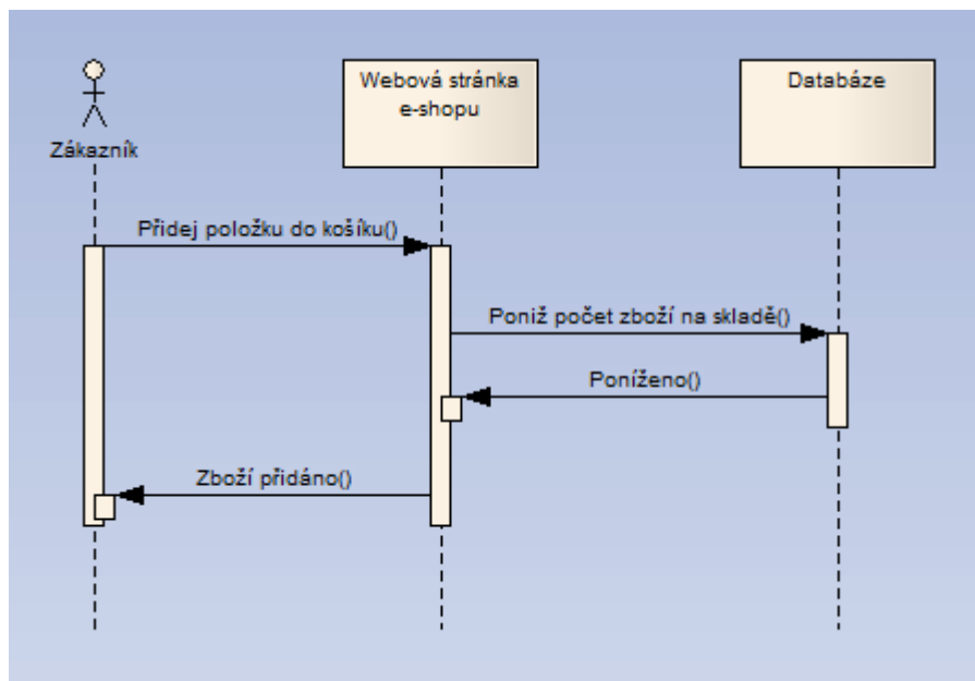
Obrázek 8 - Sekvenční diagram
