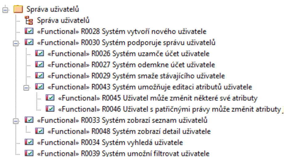
Obrázek 10 - Hierarchie požadavků
