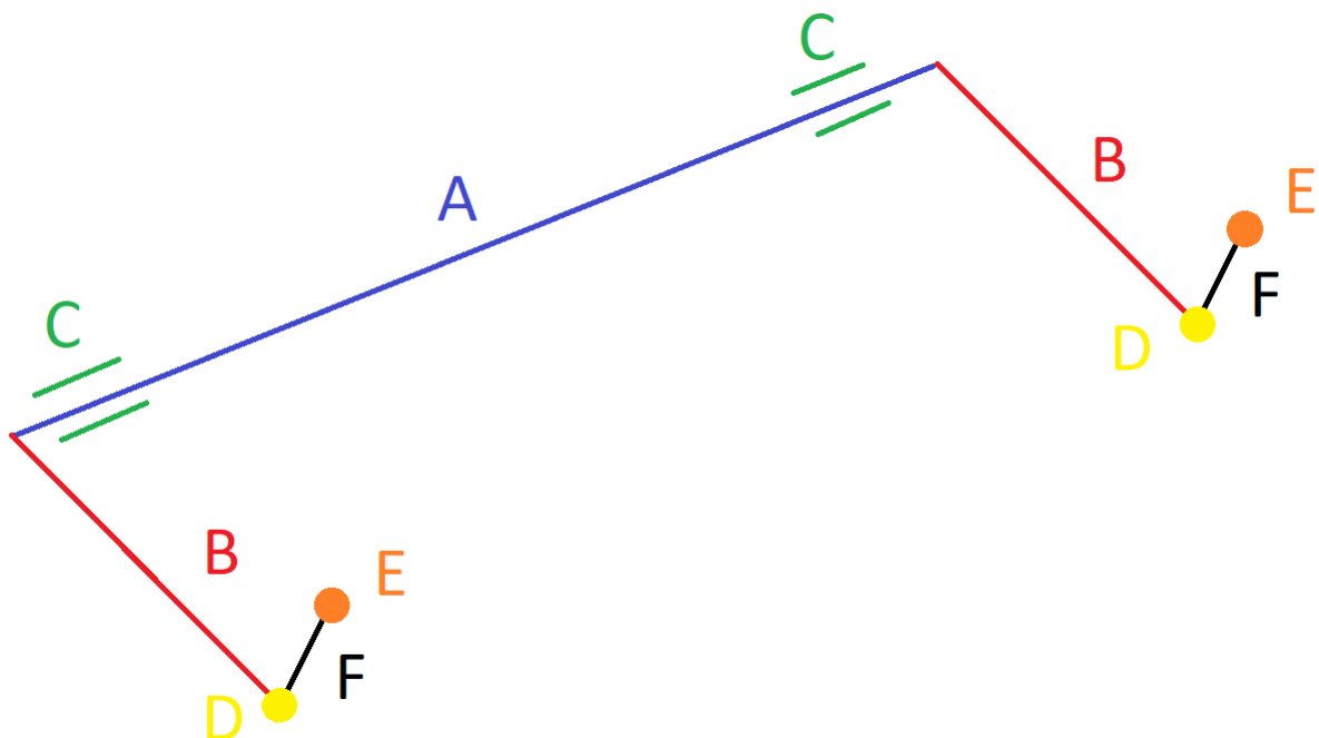
Obr. 25 Schéma zdrojů poddajnosti předního stabilizátoru
