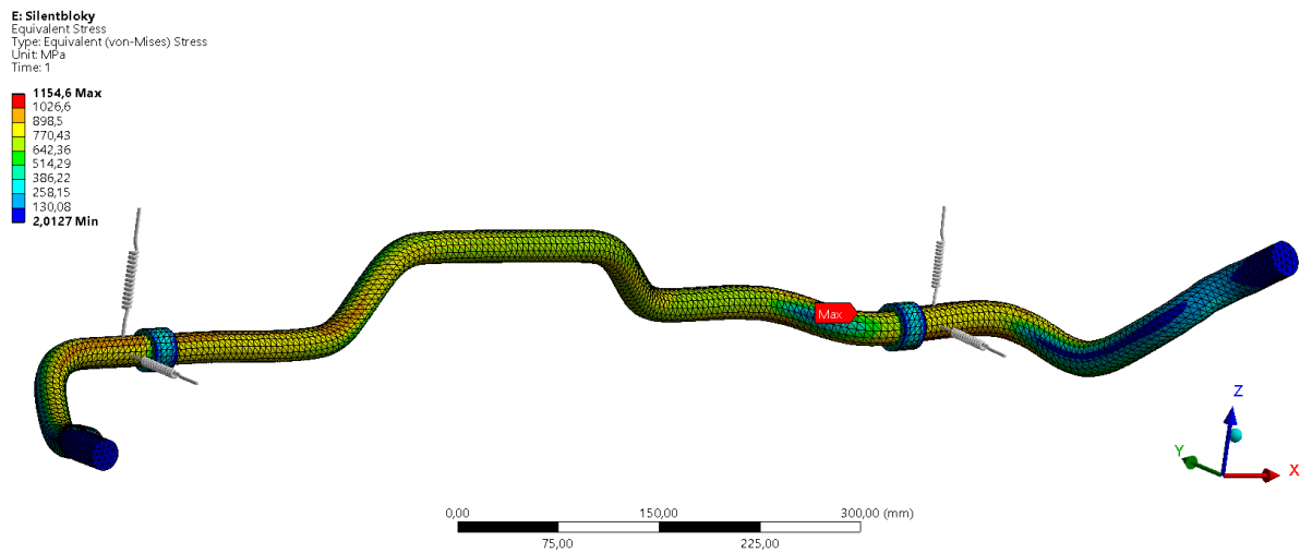
Obr. 27 Rozložení von Misesova napětí na předním stabilizátoru
