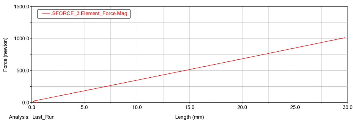
Graf 16 Závislost velikosti síly na zdvihu konce ramene vytvořená v softwaru Adams View
