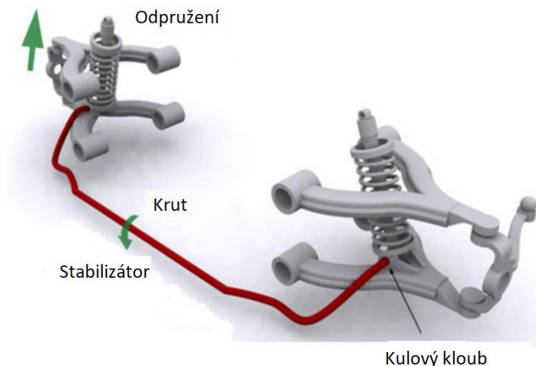
Obr. 3 Namáhání torzního stabilizátoru při zatáčení [5]
