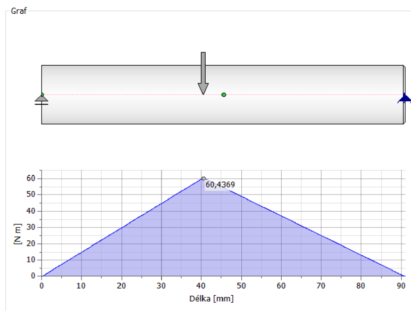
Obr. 3.16 VVU-ohybový moment
