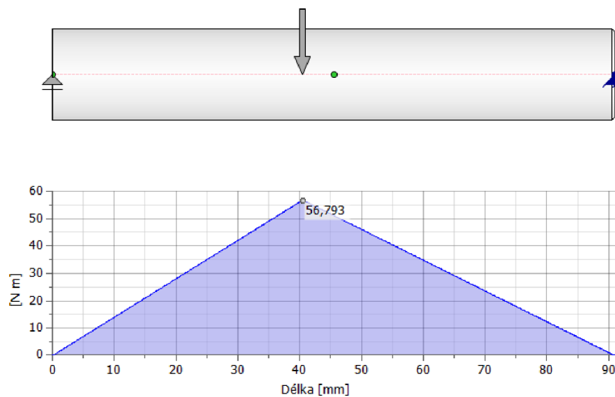
Obr. 3.18 VVU-ohybový moment
