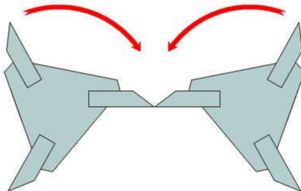
Obr. 1.6 Štěpkovací protiběžné hlavy [21]
