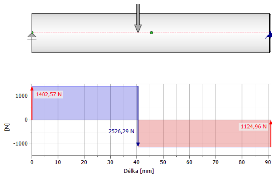
Obr. 3.17 VVU-posouvající síla
