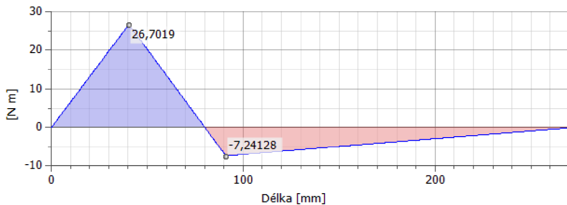
Obr. 3.20 VVU-ohybový moment
