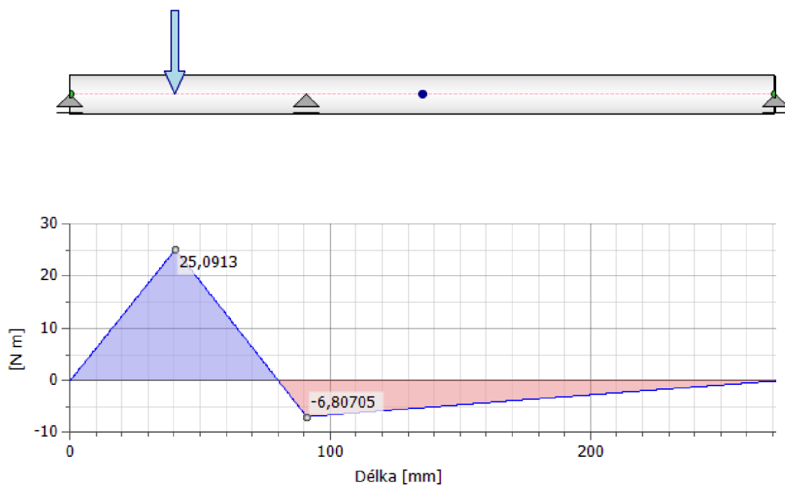
Obr. 3.22 VVU-ohybový moment
