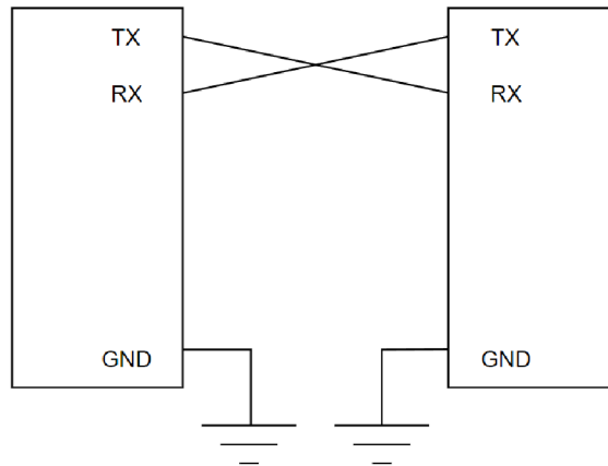
Obr. 3.1: Schéma zapojenia UART
