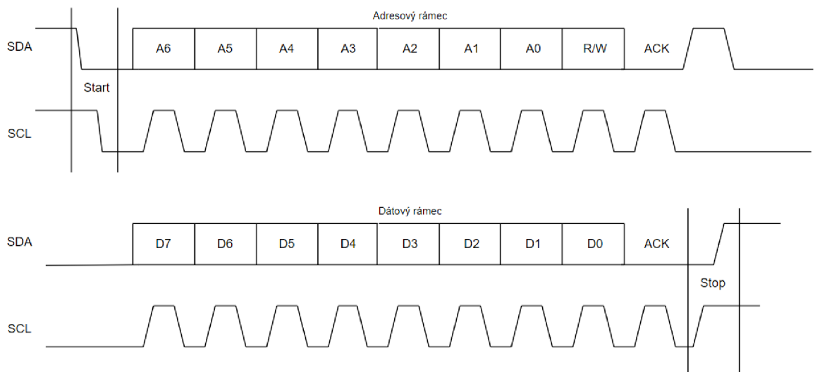
Obr. 3.4: Grafické znázornenie jedného rámca v I2C protokole
