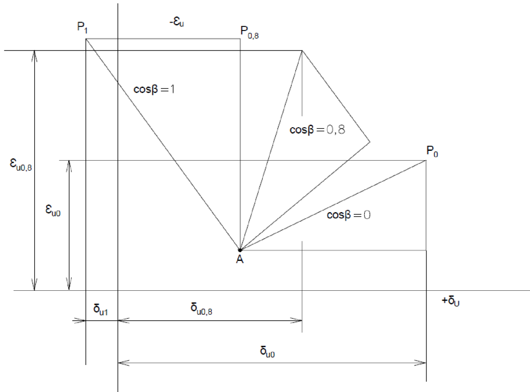
Obrázek 17 - Závislost chyb na sekundárním účinníku (převzato z [1])
