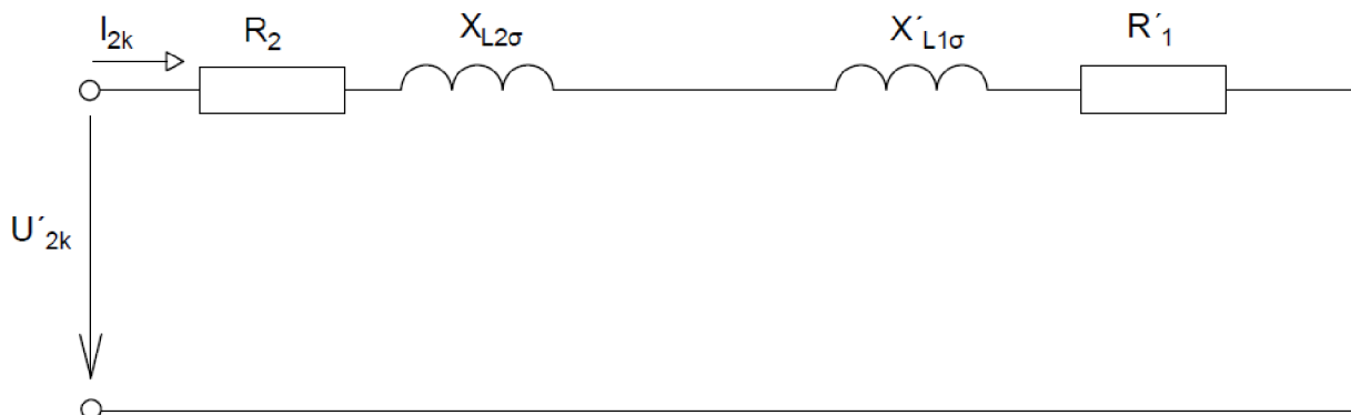
Obrázek 21 - Zjednodušené schéma zapojení transformátoru nakrátko
