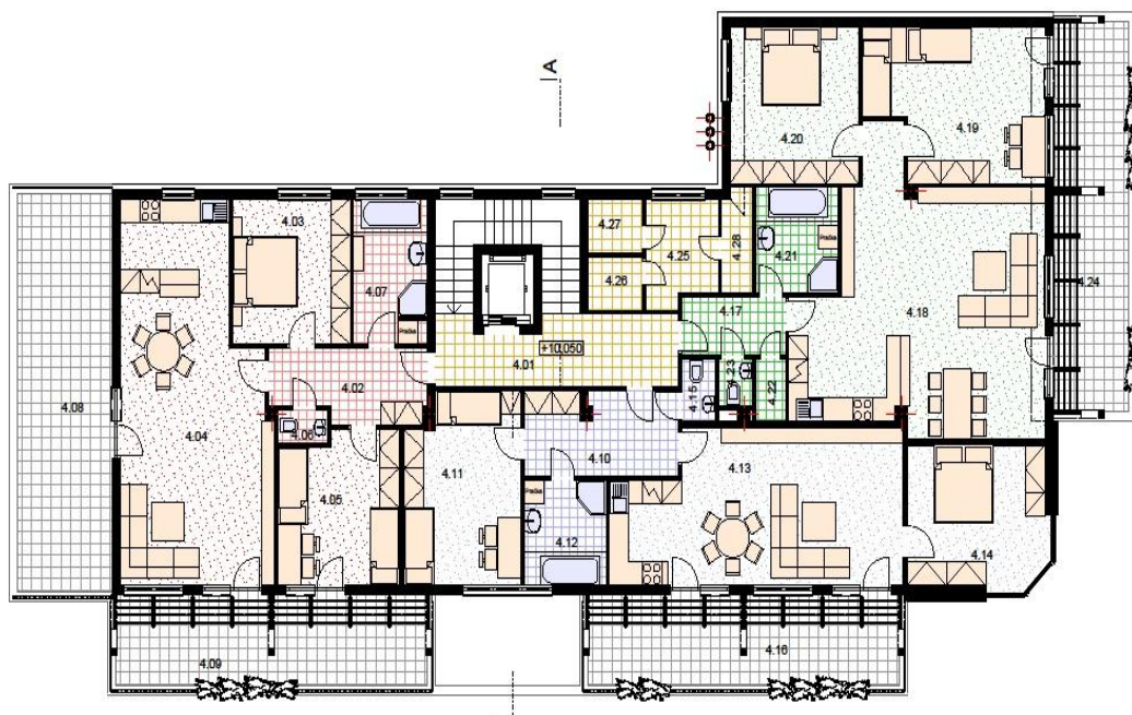
Obrázek č. 7: Půdorys 4. Nadzemního patra
