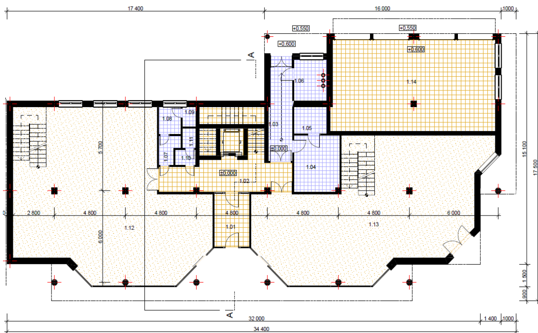
Obrázek č. 4: Půdorys 1. NP
