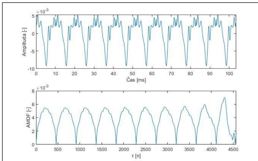
Obr. 3-3 - AMDF dokonale periodického signálu
