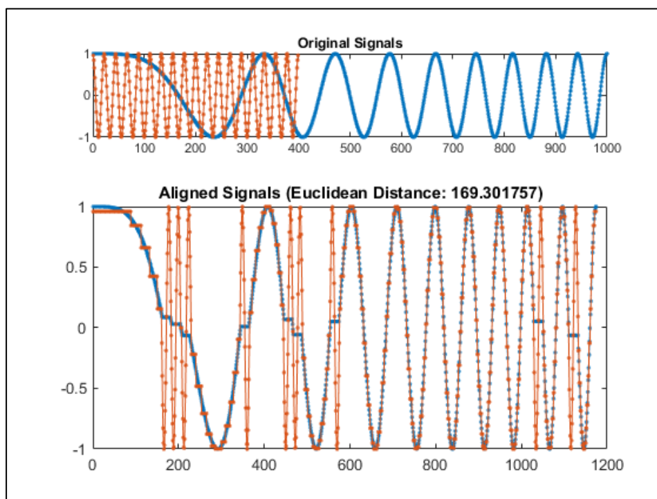
Obr. 3-5 - Znáornění roztažení funkce pomocí DTW, převzato z nápovědy MATLAB
