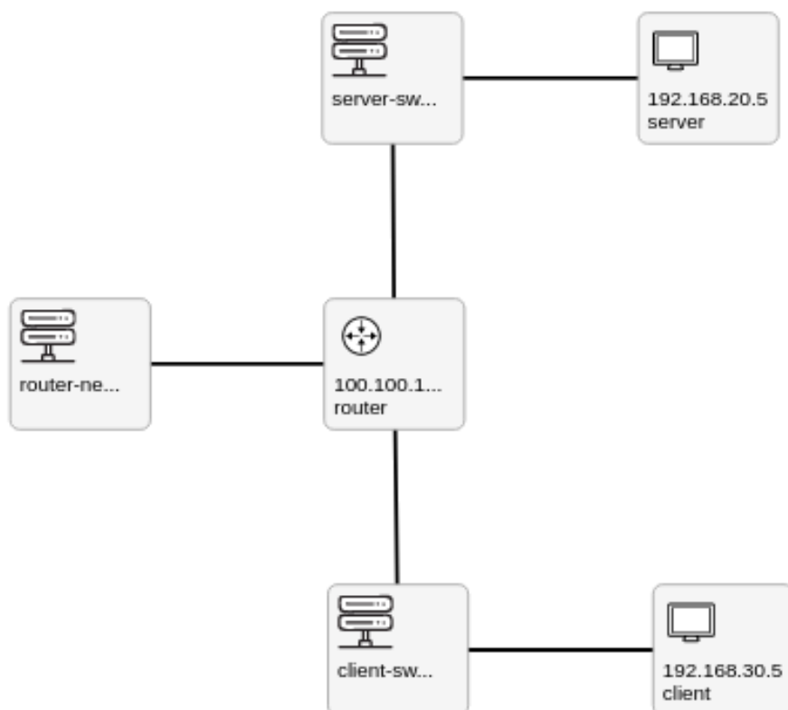
Obr. 5.6: Topologie ukázkového scénáře na platformě KYPO
