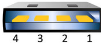
Obr. 1.1: USB-A 2.0 [5].
