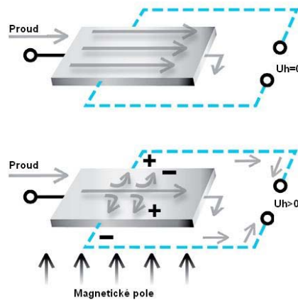
Obrázek 2.1 Názorné zobrazení funkce Hallovy sondy.
