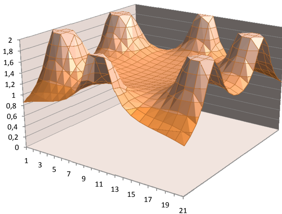
Příloha č. 5 Graf rozložení pole pro 6 Halloových snímačů, prostorový pohled.
