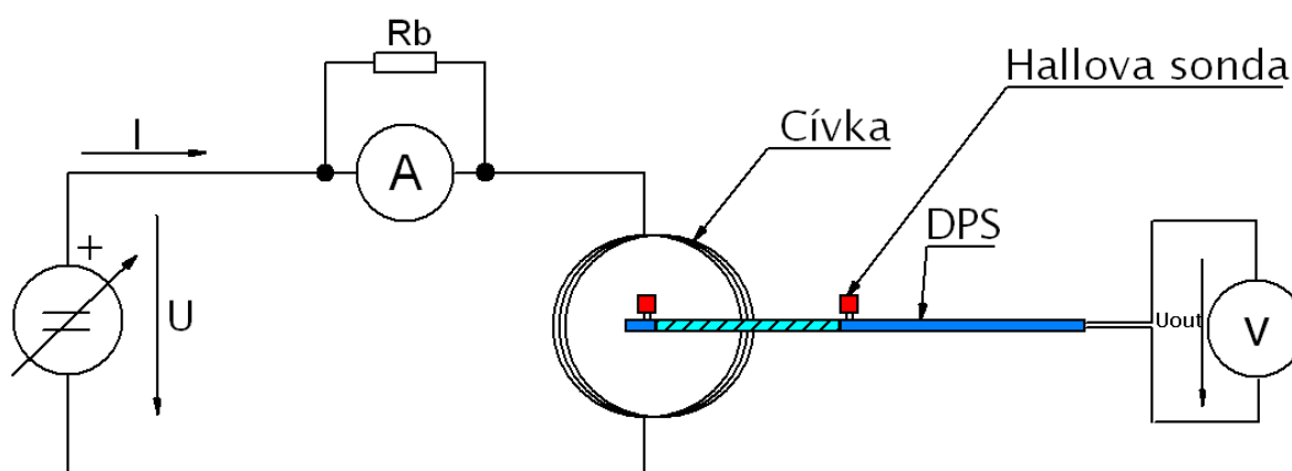
Obrázek 4.5 Schéma zapojení při měření vlastností snímače proudu.
