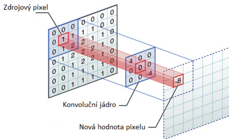
Obrázek 4.2: Princip konvoluce.
