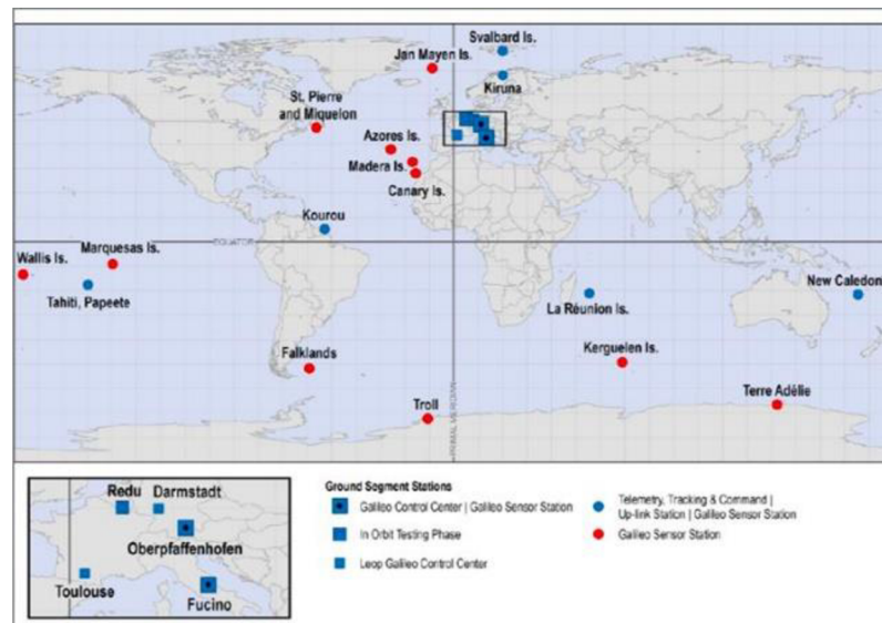
Obrázek 14: Monitorovací stanice systému Galileo [75]
