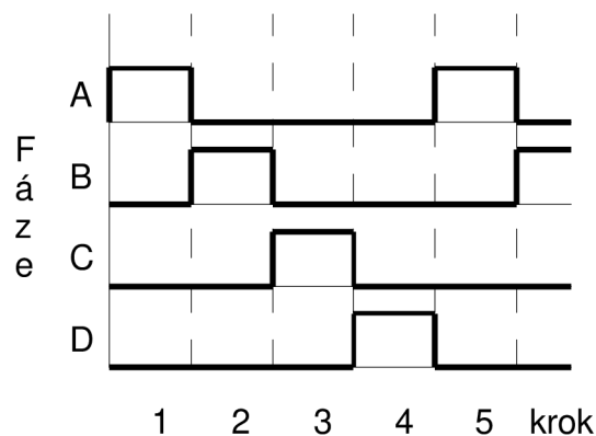
Obrázek 10: Časové průběhy čtyřtaktního řízení s magnetizací jedné fáze
