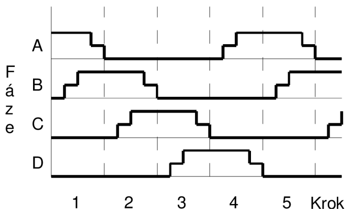
Obrázek 14: Časové průběhy při mikrokrokování – čtyřtaktní řízení s magnetizací jedné fáze
