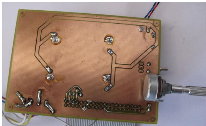
Obrázek 21: Spodní vrstva DPS měniče po realizaci
