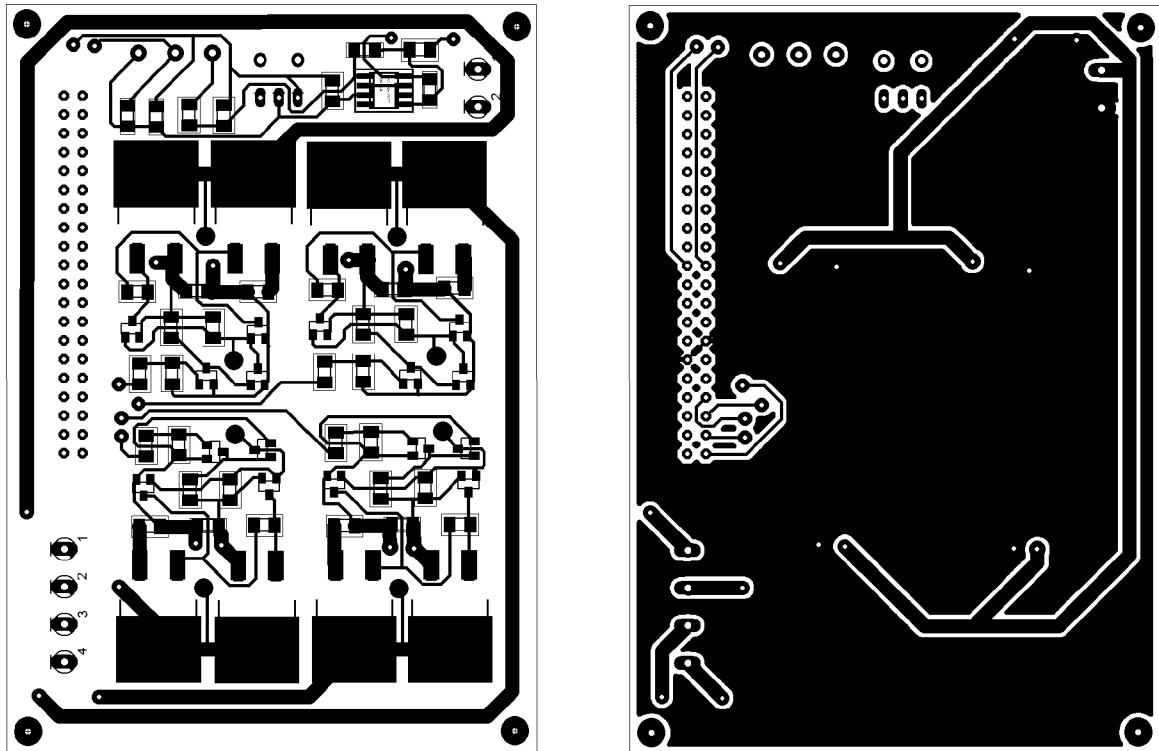
Příloha 4: Předlohy desky plošného spoje – horní vrstva (vlevo) a spodní vrstva
