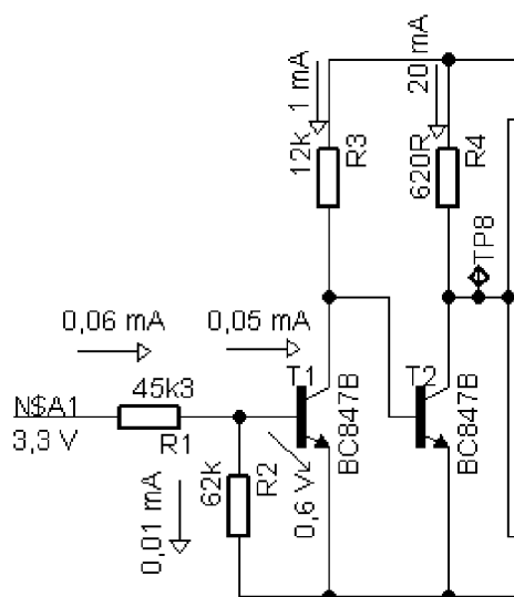
Obrázek 19: Rozložení proudů a úbytků napětí v budícím obvodu – výřez schématu
