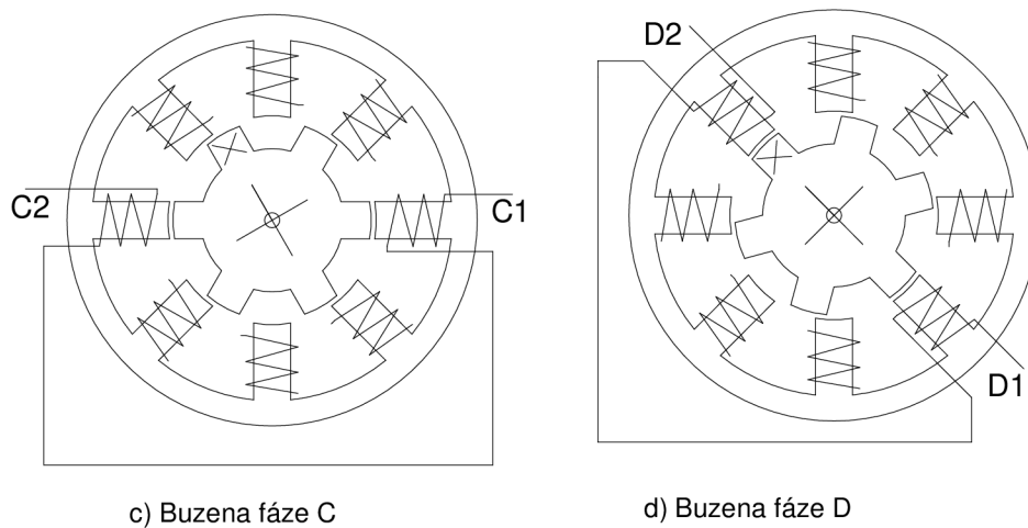
Obrázek 9: Čtyřtaktní řízení čtyřfázového KM s magnetizací jedné fáze – 4 kroky
