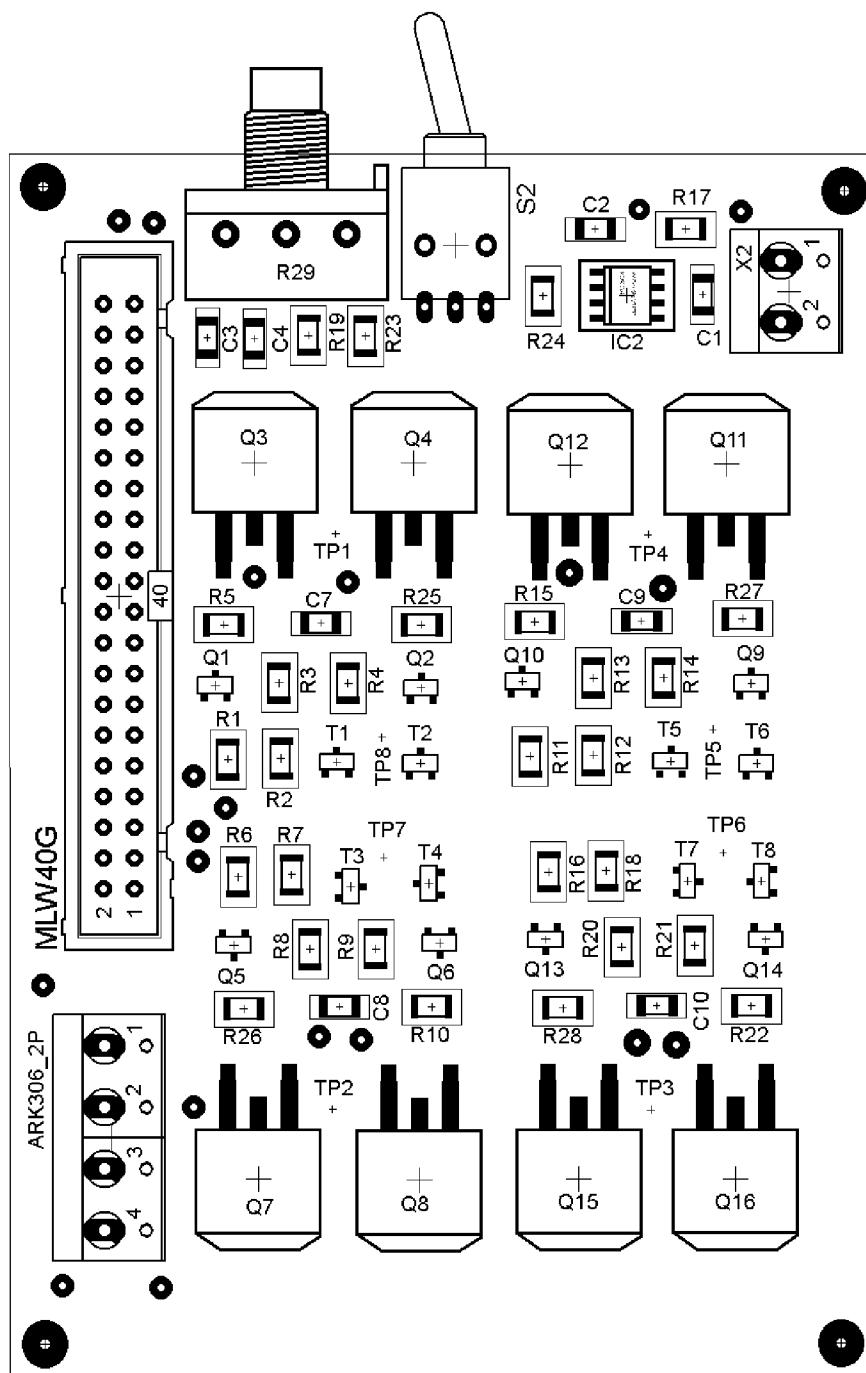
Příloha 3: Osazovací plán desky plošného spoje
