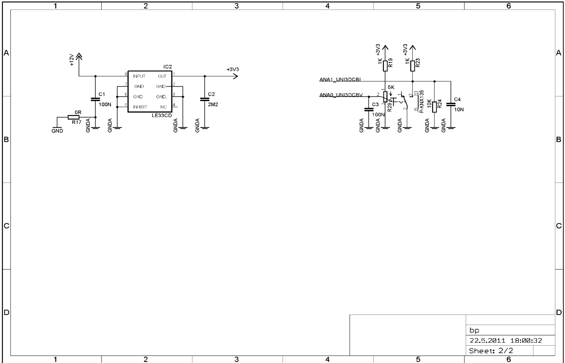
Příloha 2: Schéma zapojení – napájecí a ovládací část
