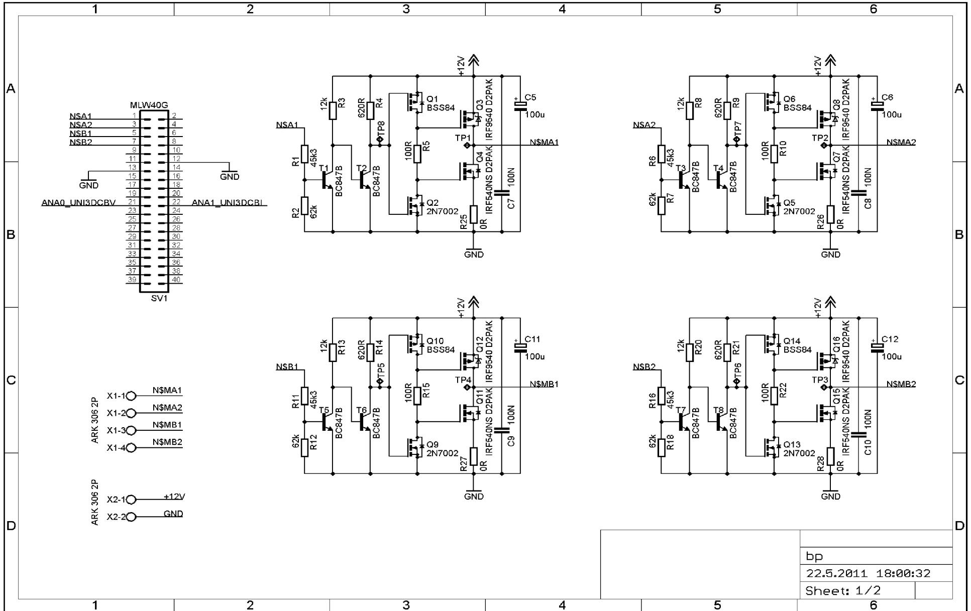
Příloha 1: Schéma zapojení – budící část
