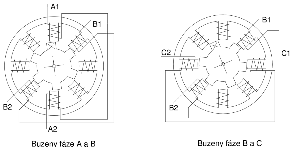
Obrázek 11: Čtyřtaktní řízení čtyřfázového KM s magnetizací dvou fází – dva kroky
