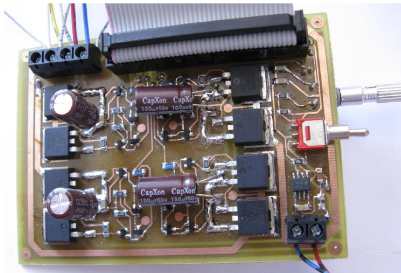
Obrázek 20: Horní vrstva DPS měniče po realizaci
