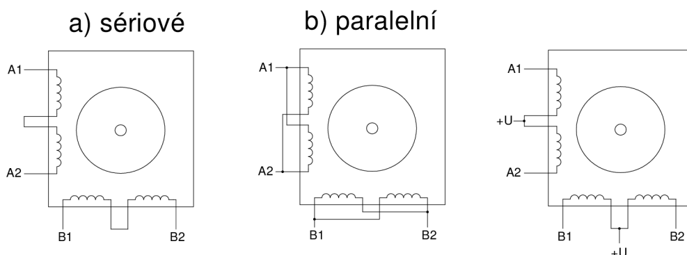
Obrázek 8: Možné způsoby zapojení dvoufázového hybridního KM
