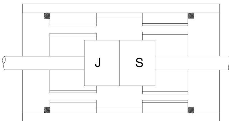
Obrázek 6: Konstrukční uspořádání KM s axiálně polarizovaným magnetem v řezu
