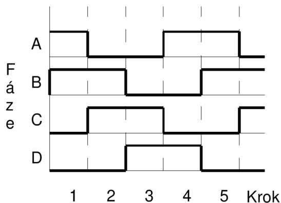
Obrázek 12: Časové průběhy čtyřtaktního řízení s magnetizací dvou fází
