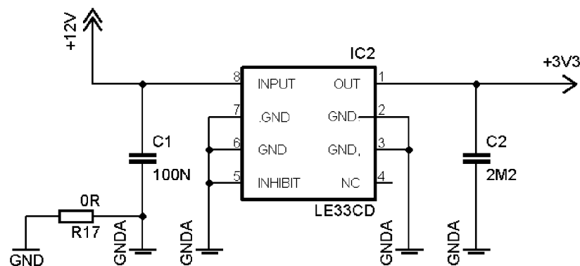
Obrázek 17: Zapojení stabilizátoru LE33CD pro napětí 3,3V
