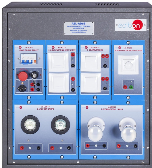
Obrázek 2.3: Edibon - řízení svítivosti [9]
