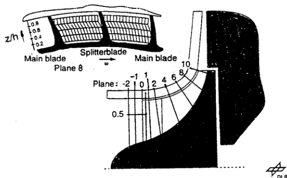
Obr. 2.7 Označení rovin pro laserová měření, převzato z Eisenlohr et al. [12]
