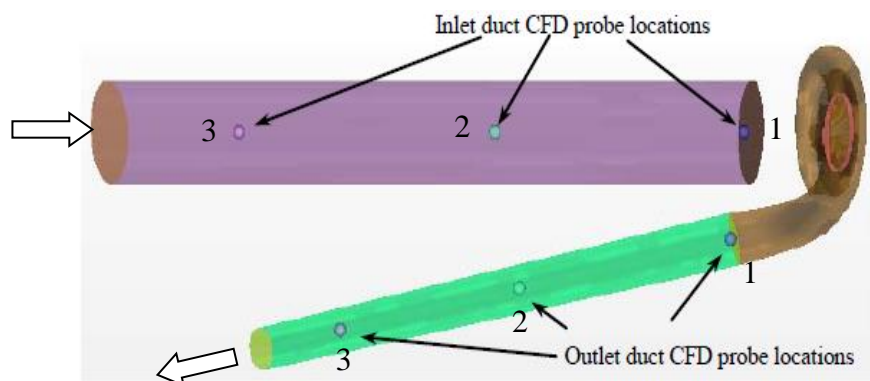
Obr. 3.18 Model měřicí soustavy odstředivého kompresoru, převzato z Mendonca et al. [23]
