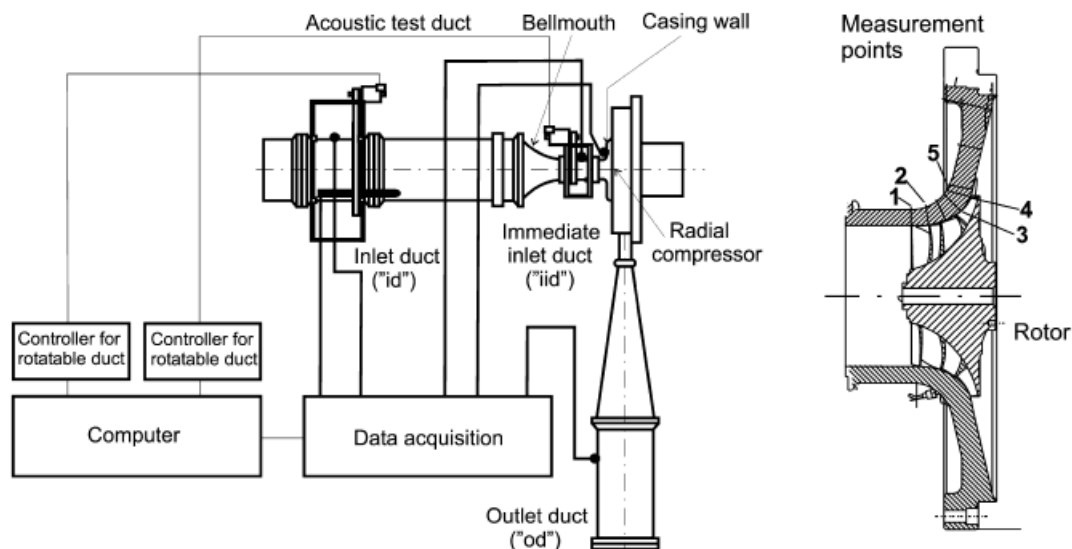
Obr. 3.6 Detail měřící soustavy a rotoru s odběrem tlaků ze skříně, převzato z Raitor a Niese [19].
