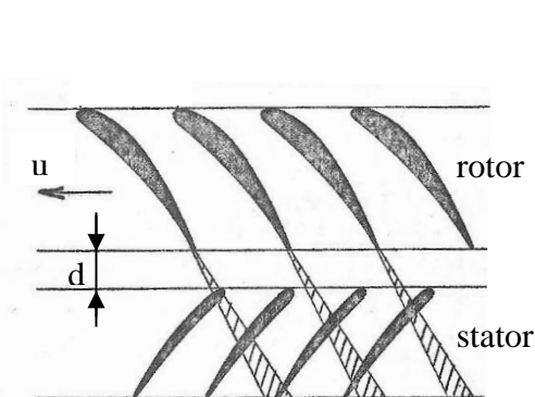
Obr. 3.40 Úplav za rotorovou mříží stupně axiálního kompresoru, převzato z Šulc [20]
