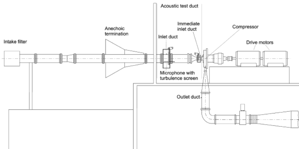
Obr. 3.5 Schéma měřící tratě v DLR institutu, převzato z Raitor a Niese [19]
