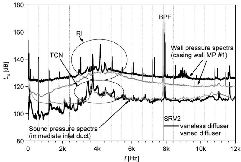
Obr. 3.10 Měření tlakových spekter ve vstupním kanále a na skříní kompresoru v místě MP #1, pro kompresor SR V2, při n_{red} = 36\,000\text{ min}^{-1} na pracovní čáře při konstantním nastavení škrticí klapky, převzato z Raitor a Niese [19]
