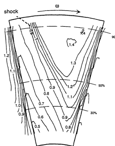
Obr. 2.8 Rozložení Machových čísel v rovině 0, převzato z Eisenlohr et al. [12]
