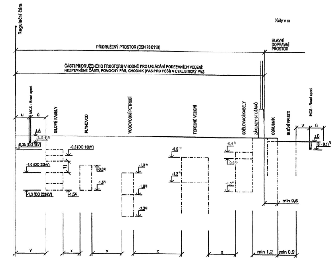
Obrázek 44 Prostorové uspořádání 92
