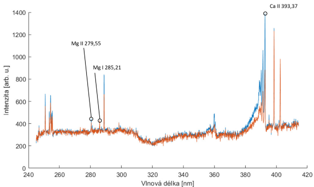
Obrázek 4.19: Vybraná spektra myší kosti s vyznačenými spektrálními čárami.
