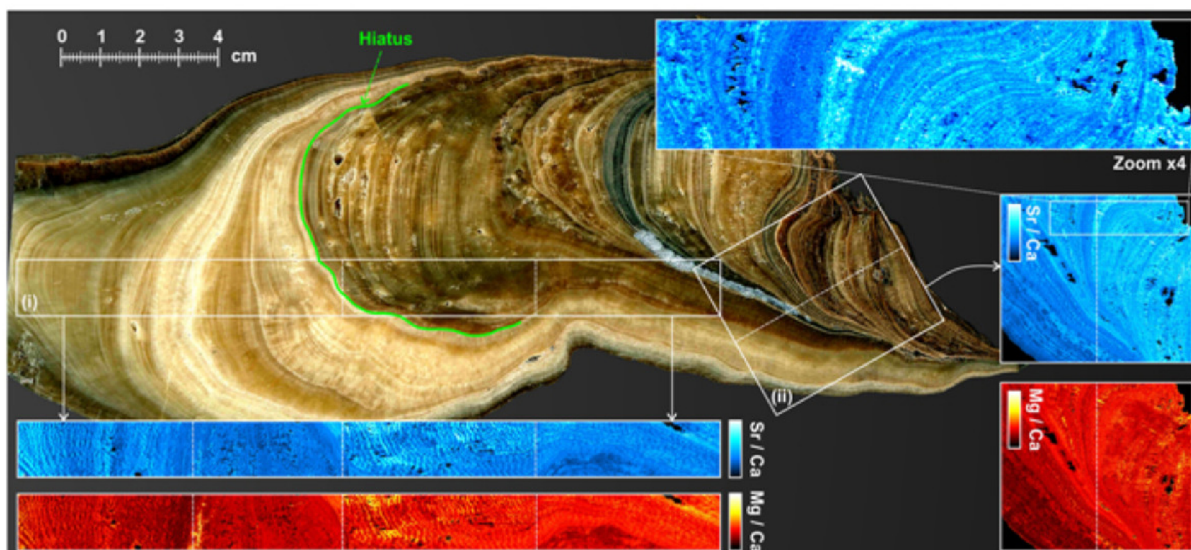
Obrázek 3.3: Příklad elementárních map jeskynního krápníku. „Hiatus” reprezentuje šterbinu způsobenou růstem krápníku v čase. Převzato z [56].
