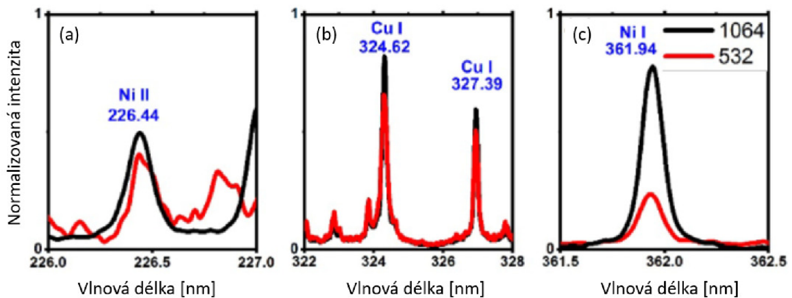
Obrázek 2.4: Porovnání emisních spekter pro dvě vlnové délky laseru. Převzato z [50].
