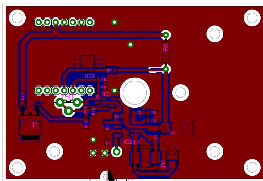
Obr. E.1: Výkres desky plošných spojů řídicího obvodu laserové diody - horní vrstva
