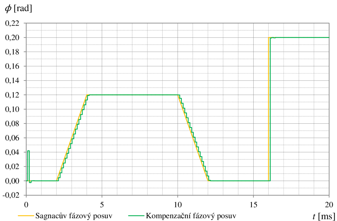
Obr. C.5: Simulovaný průběh kompenzace Sagnacova fázového posuvu
