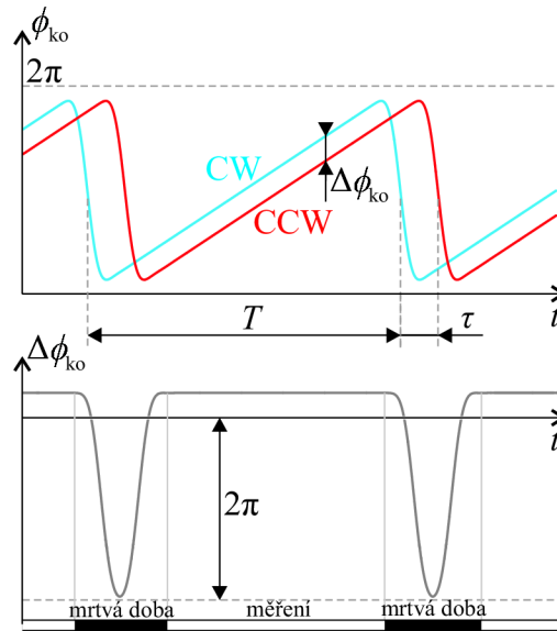
Obr. 4.11: Použití filtrace u pilovité fázové modulace pro kompenzaci rotace
