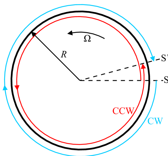
Obr. 1.1: Vliv úhlové rychlosti \Omega na optické dráhy paprsků [6]
