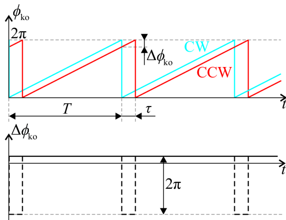
Obr. 2.9: Průběh kompenzačního fázového posuvu [6]
