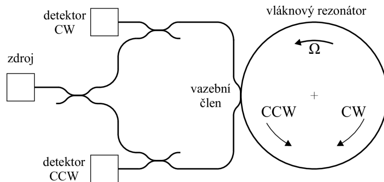
Obr. 3.3: Schéma reciprokého uspořádání R-FOG [3]; upraveno
