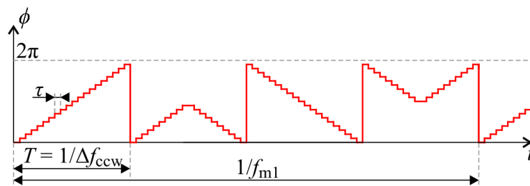
Obr. 3.7: Průběh hybridní pilovité modulace frekvence [44]; upraveno
