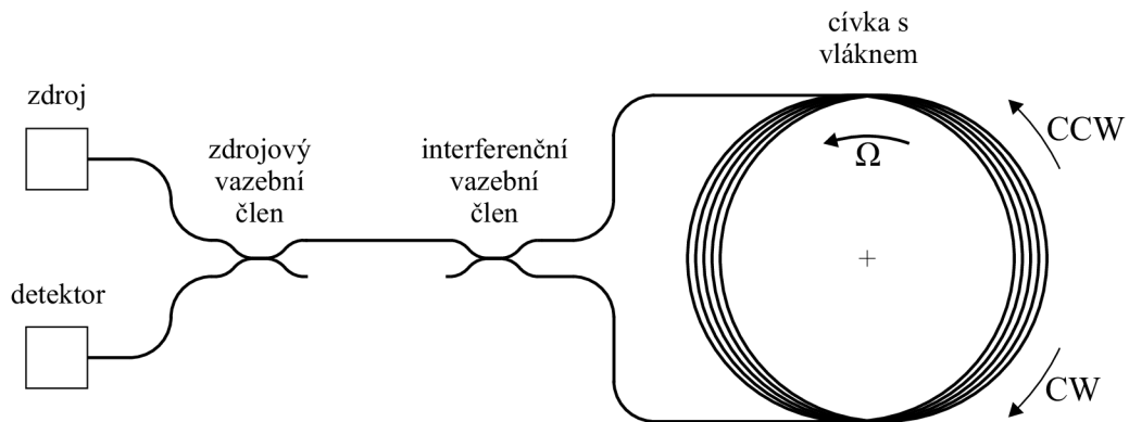
Obr. 2.3: Schéma reciprokého uspořádání I-FOG [6]
