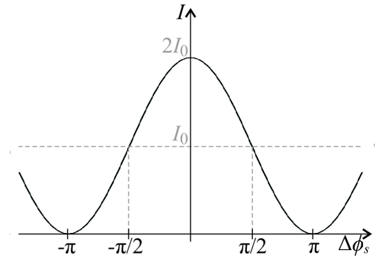
Obr. 2.2: Závislost výstupní intenzity na fázovém posuvu [6]
