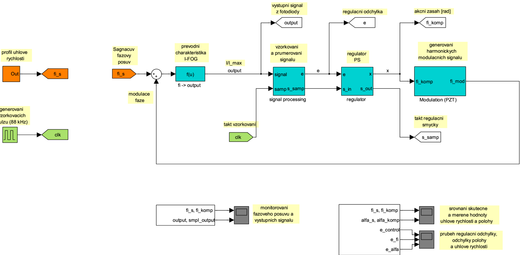
Obr. C.7: Simulační schéma I-FOG a zpracování signálu pro návrh regulační smyčky
