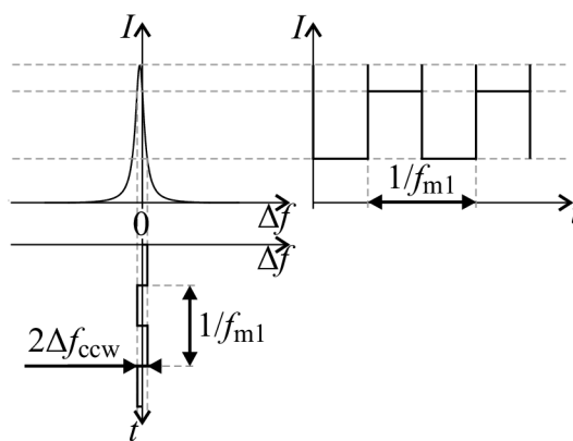
Obr. 3.9: Průběh frekvence a intenzity signálu otevřené smyčky při f_{ccw} \neq f_0 [50]; upraveno
