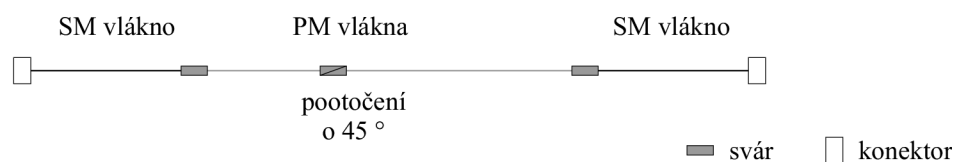
Obr. 4.3: Schéma vláknového Lyotova depolarizátoru
