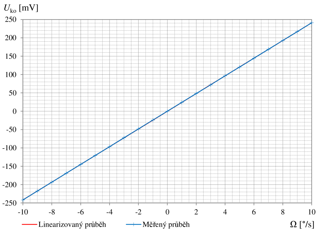
Obr. 5.4: Graf závislosti kompenzačního napětí na úhlové rychlosti U_{ko}(\Omega) na rozsahu \pm 10 °/s
