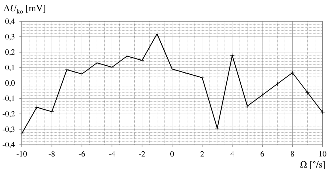
Obr. 5.5: Graf závislosti chyby linearity kompenzačního napětí na úhlové rychlosti \Delta U_{ko}(\Omega) na rozsahu \pm 10 °/s
