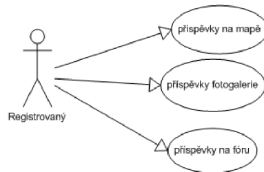
Obrázek 4.3: Registrovaný uživatel
