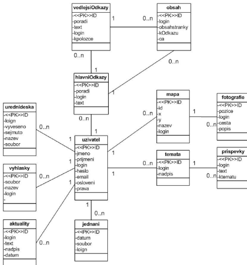
Obrázek 4.1: ER diagram
