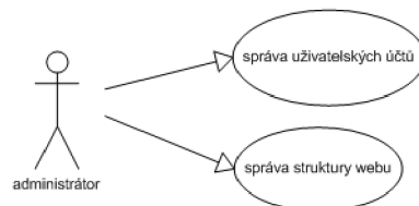
Obrázek 4.5: Adminitrátor
