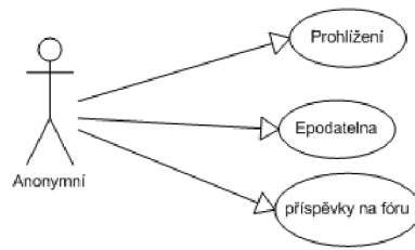
Obrázek 4.2: Anonymní uživatel
