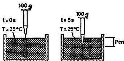
Obrázek 3- 10: Princip penetrace, [8]
