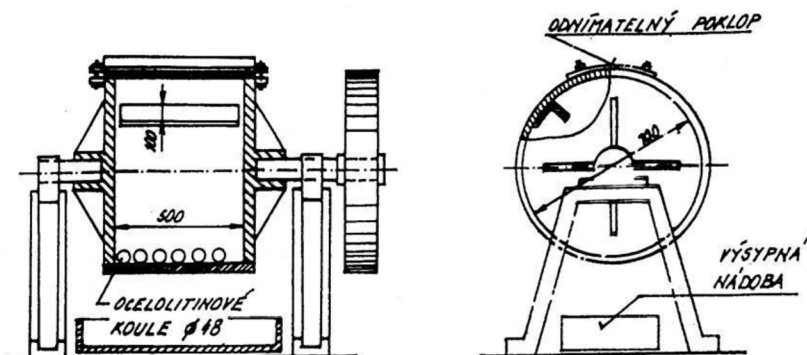
Obrázek 3- 9: Otlukový buben pro zkoušku Los Angeles, [6]
