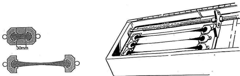
Obrázek 3- 16: Princip vratné duktility, [8]
