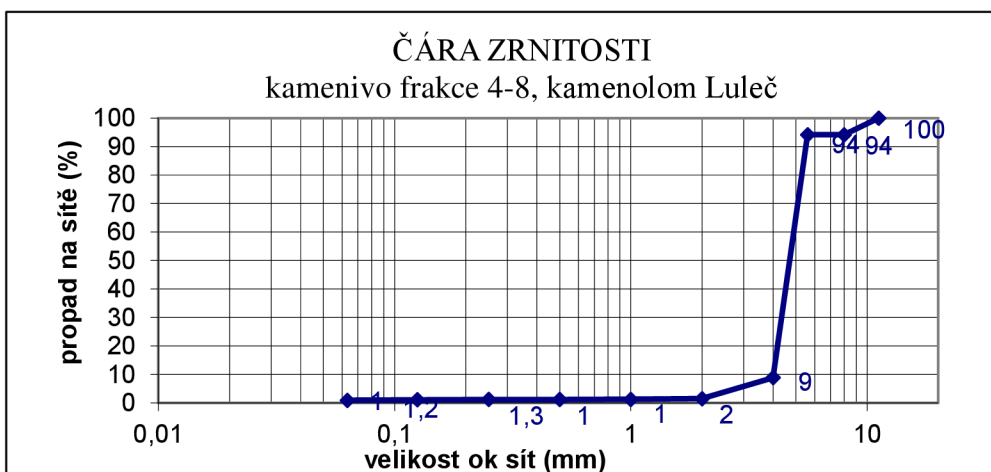
Graf 3- 3: Čára zrnitosti frakce 4/8
