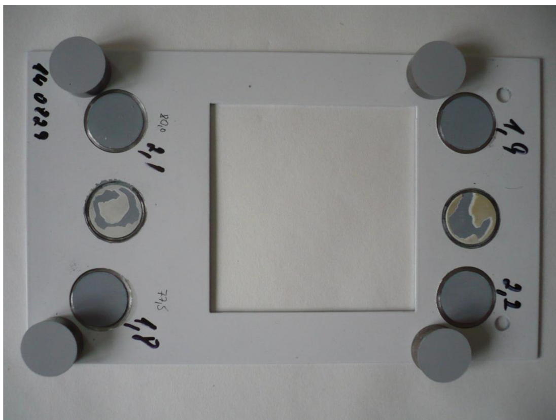
Obr. 24 Vzorek L3 po odtrhové zkoušce
