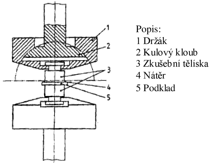
Obr. 14 – Schéma trhacího zařízení [6]
