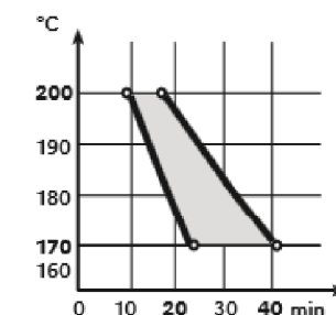
Objektová teplota versus vypalovací čas
