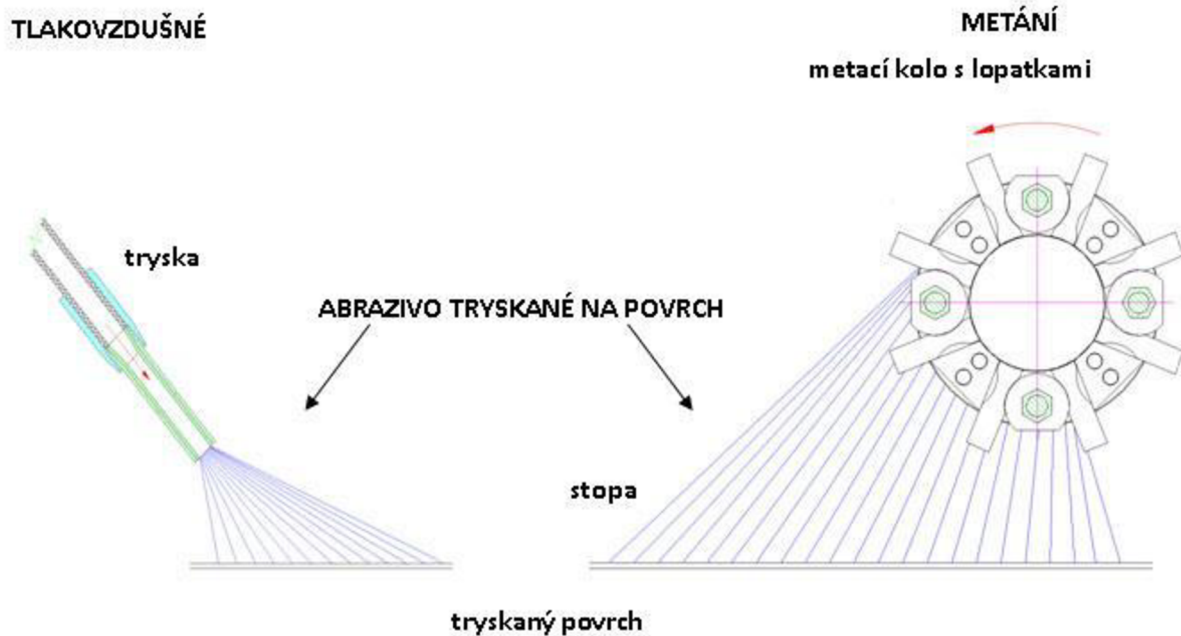
Obr. 9 Způsoby otryskávání [20]
