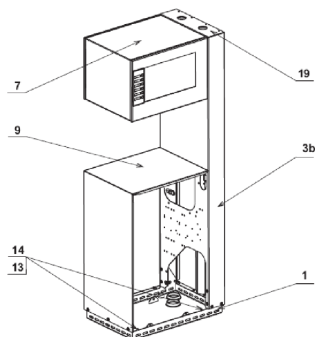
Obr. 6 Schéma skeletu [1]
