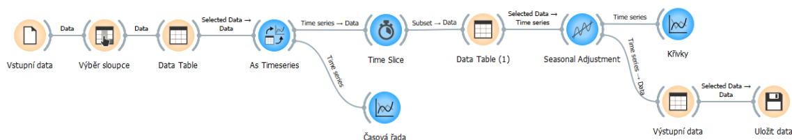
Obr. 20 Model využitý pro dekompozici časových řad
