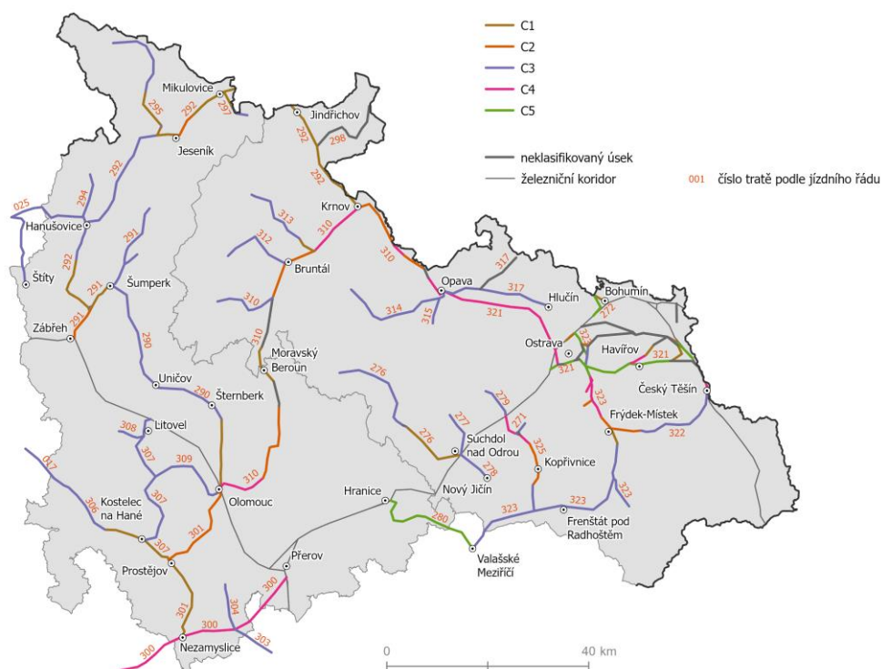
Obr. 52 Výsledky shlukování podle průběhu počtu nákladních vlaků v letech 2016–2019
