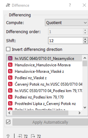
Obr. 18 Nastavení parametrů uzlu Difference
