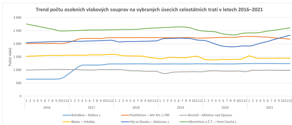
Obr. 21 Příklad výsledného grafu po dekompozici časových řad
